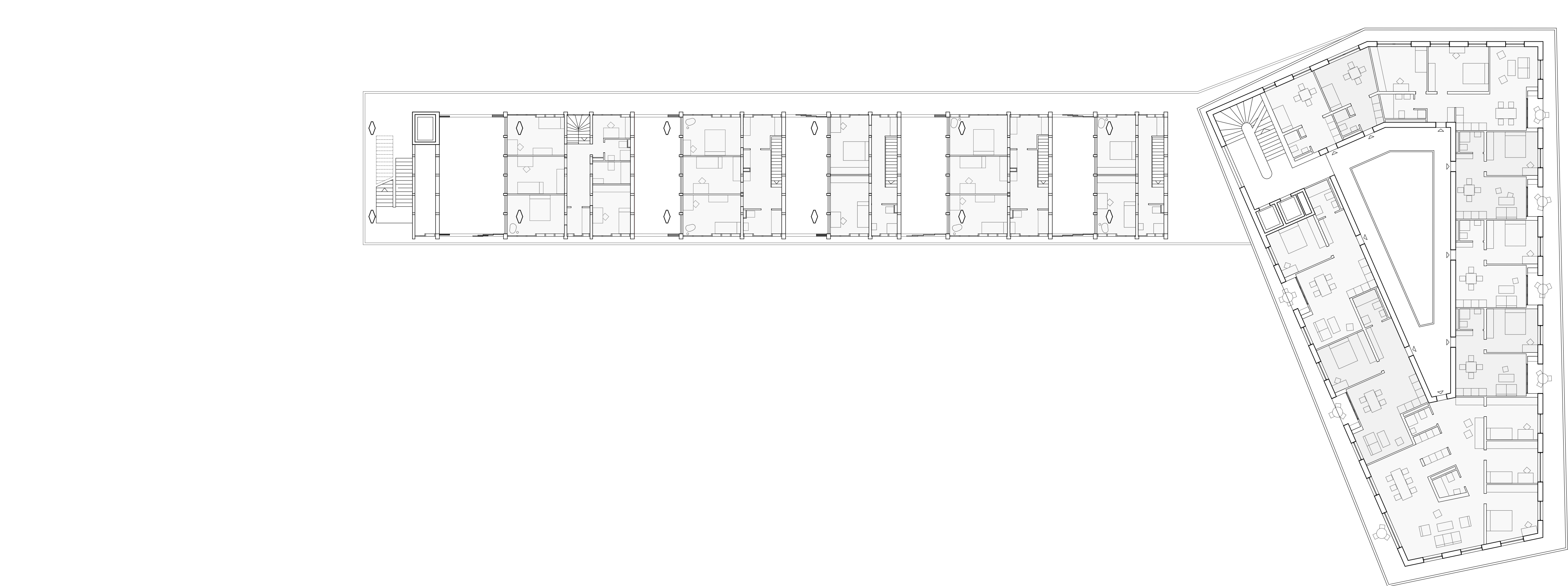
Plan 2 ème étage 1. 200 ème
