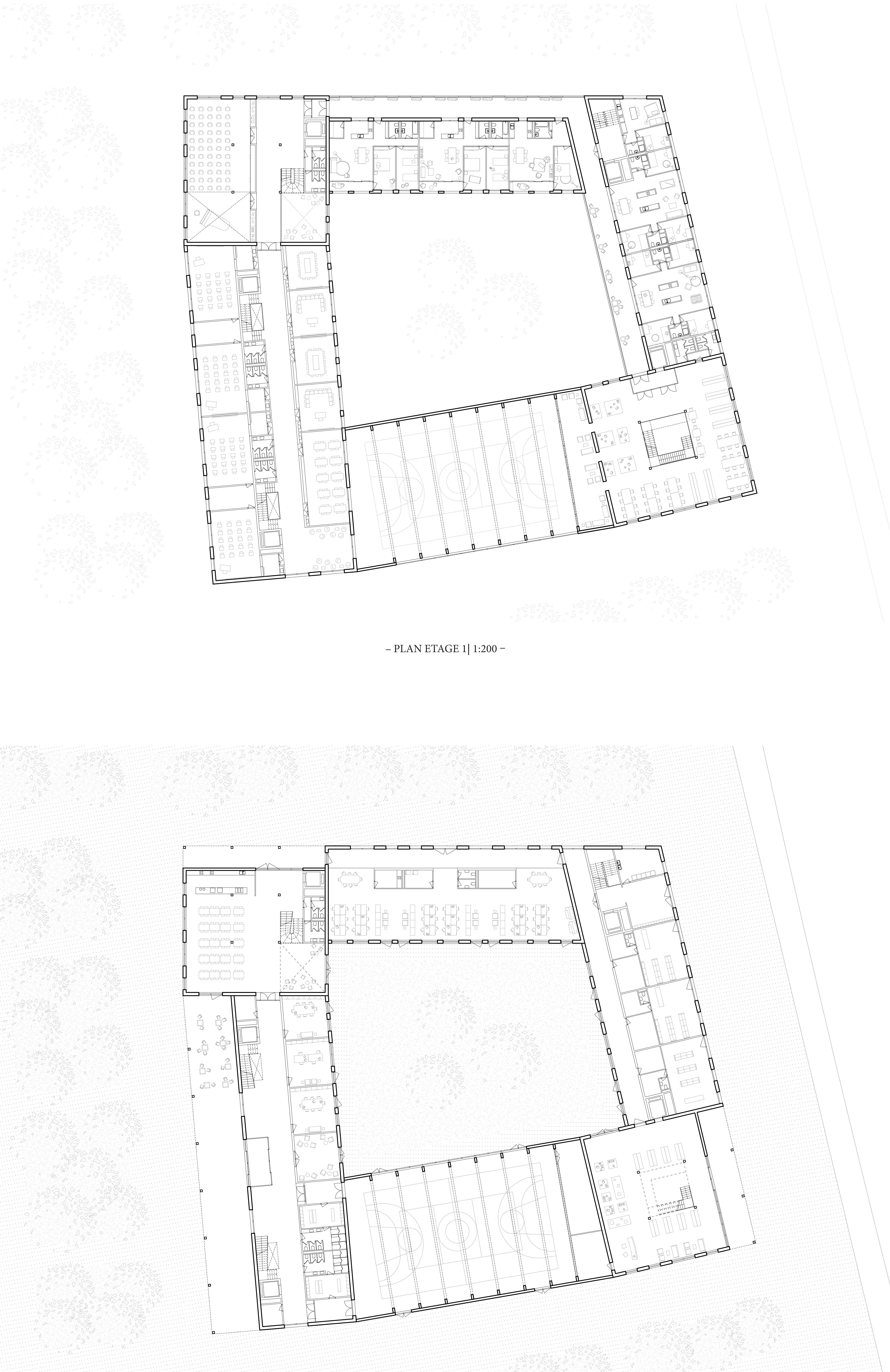
- PLAN REZ-DE-CHAUSSEE | 1:200 -
