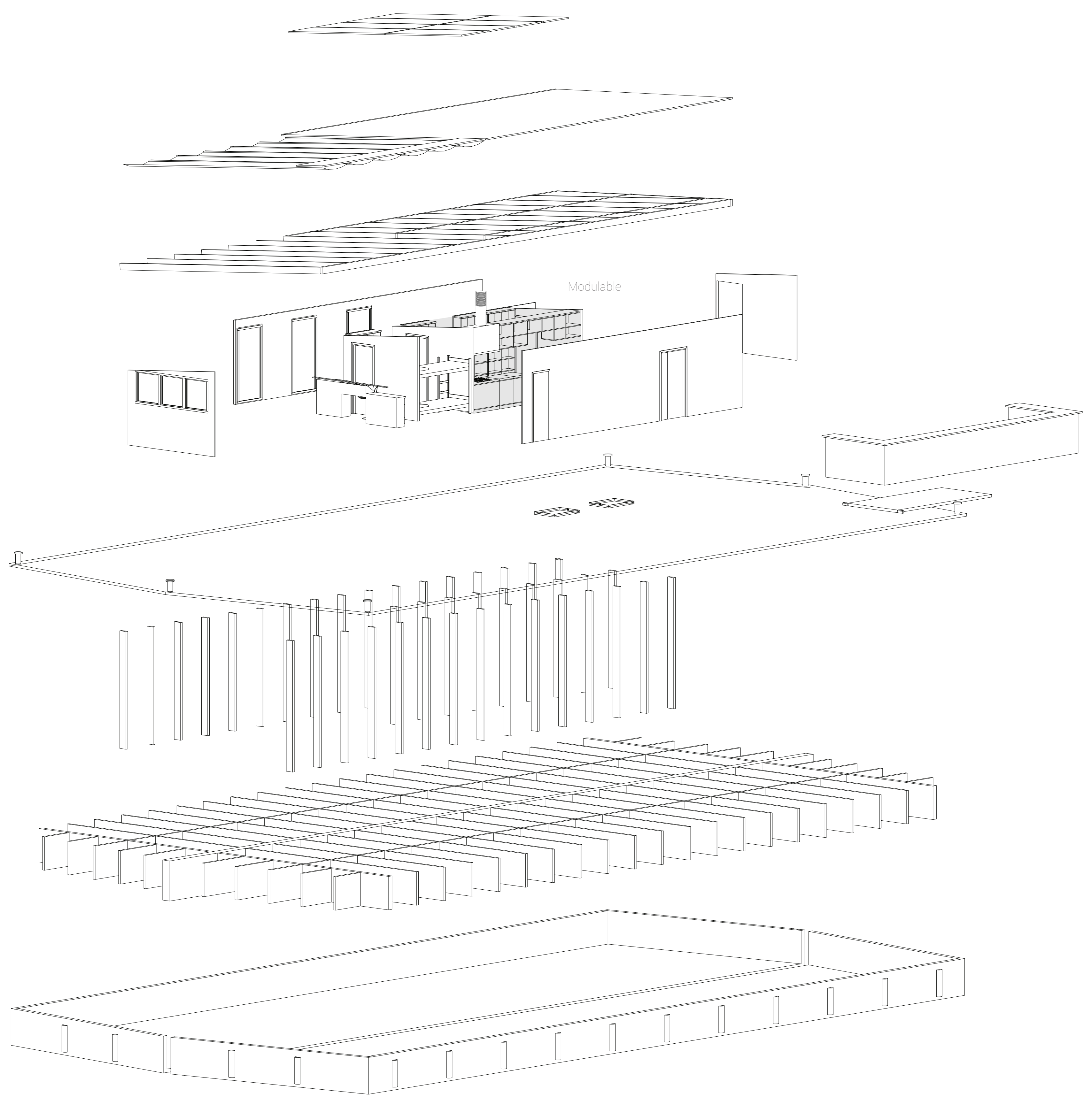
Axonométrie constructive
