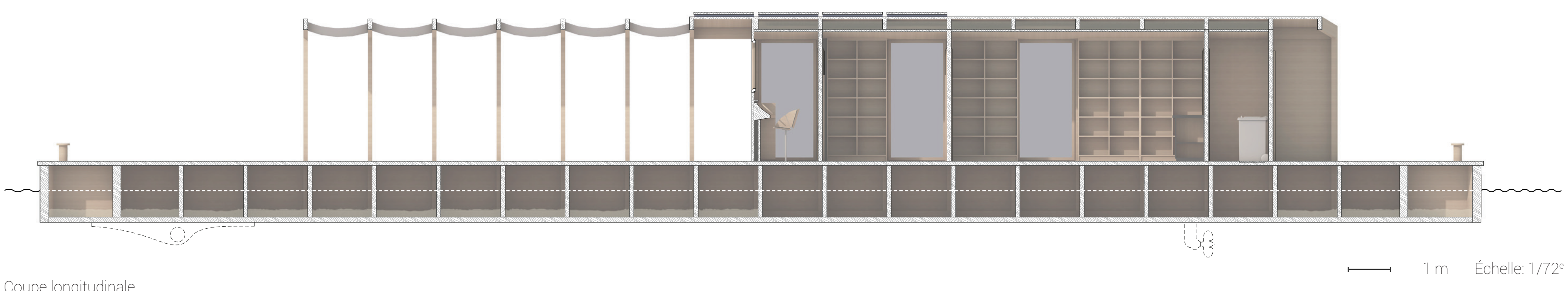
Coupe longitudinale 1 m Échelle: 1/72 e
