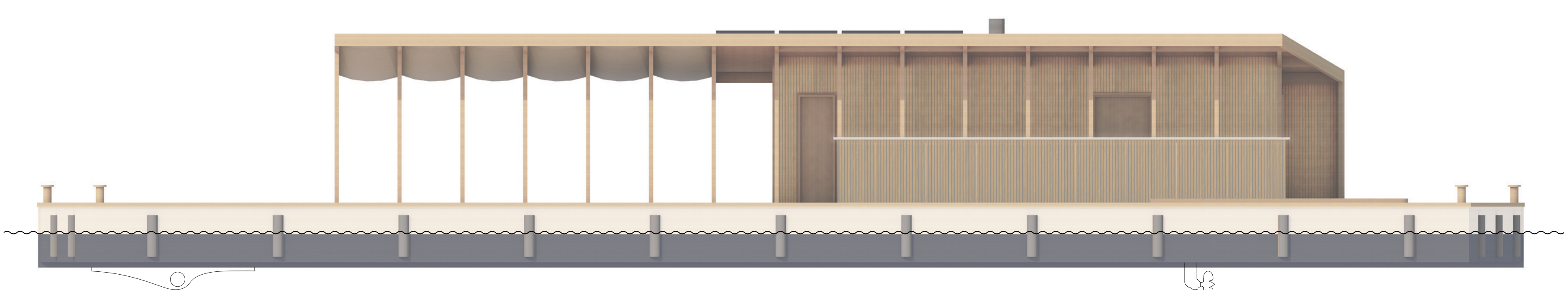
Élévation longitudinale 1 m Échelle: 1/72 e
