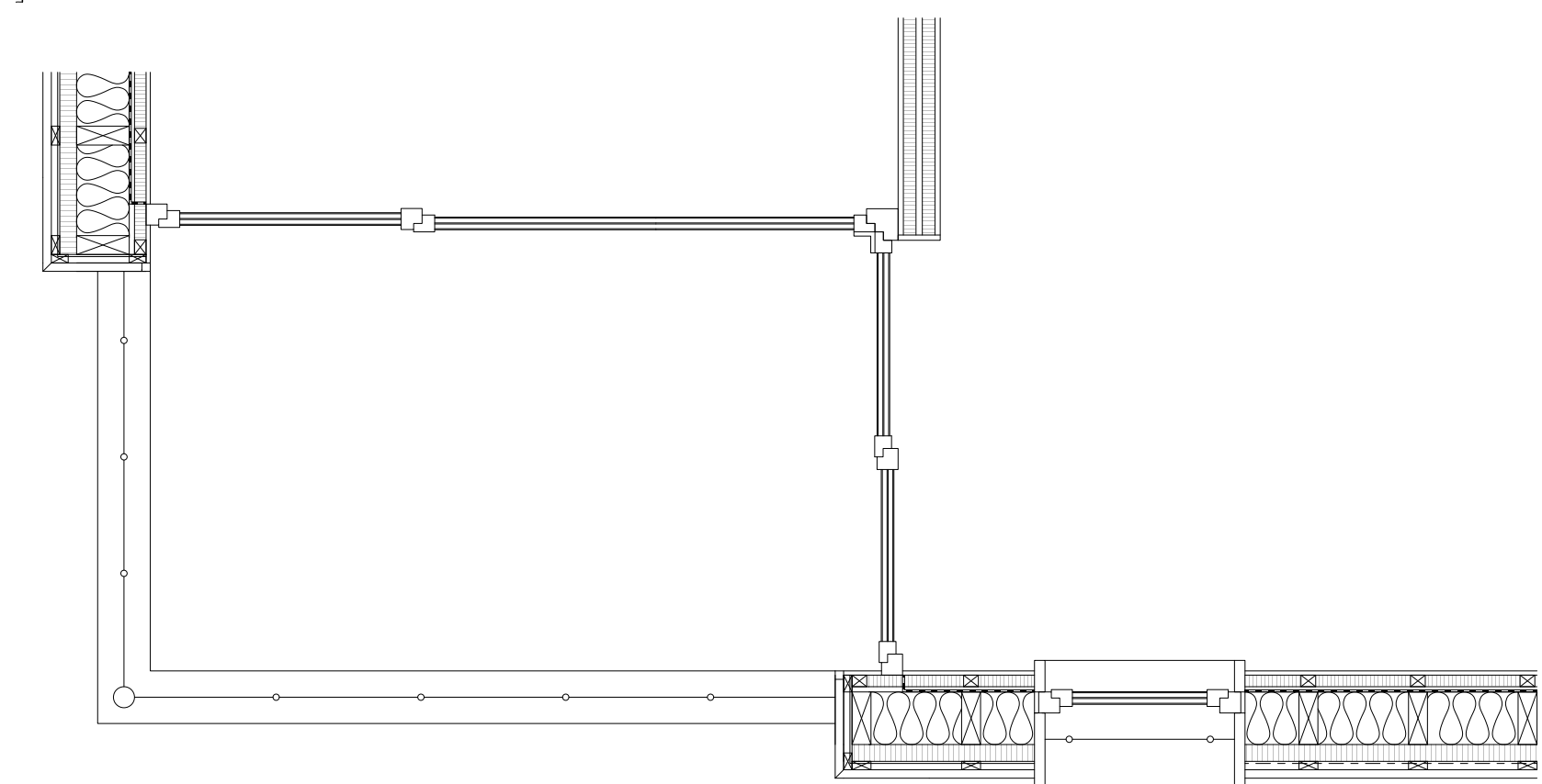
Détail constructif 1:33
