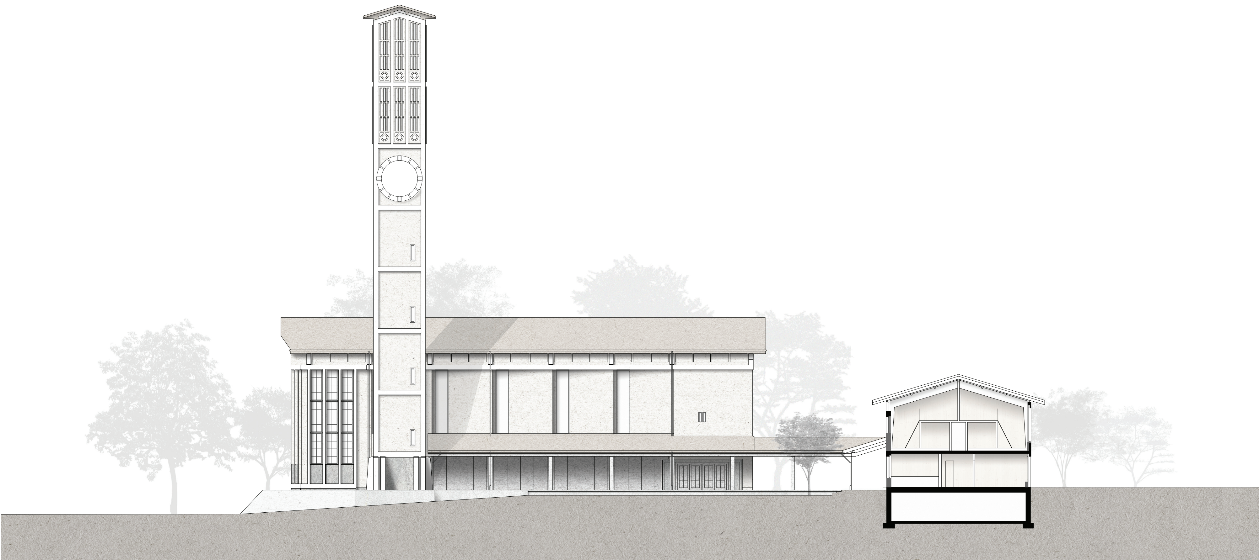
Coupe AA' 1:200
