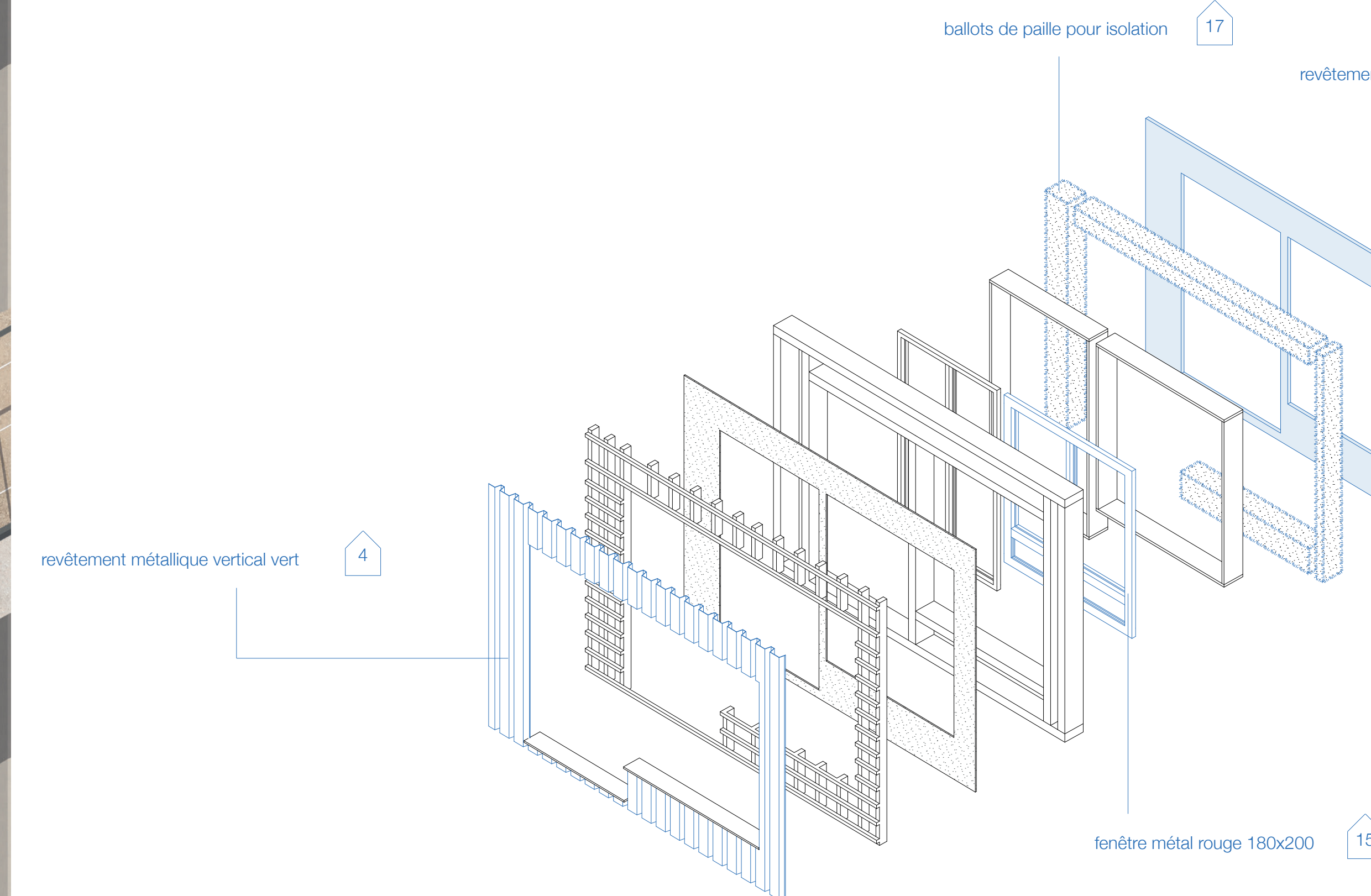
principe de façade échelle 1:50
