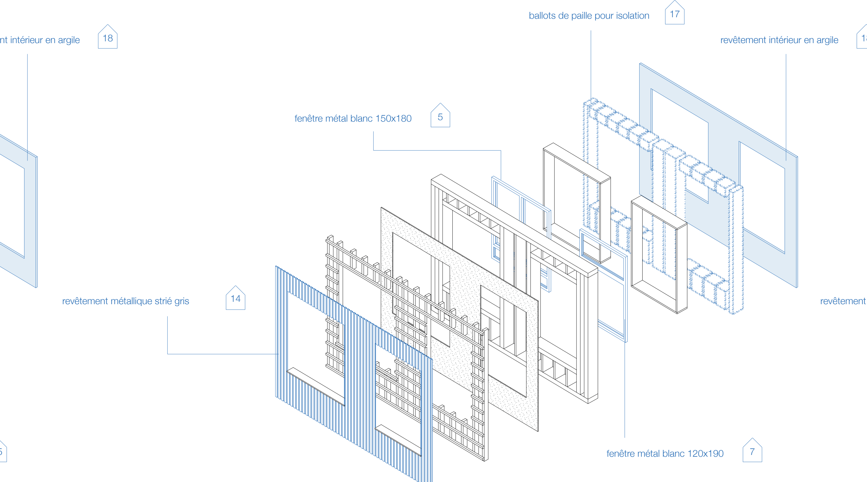
principe de façade échelle 1:50
