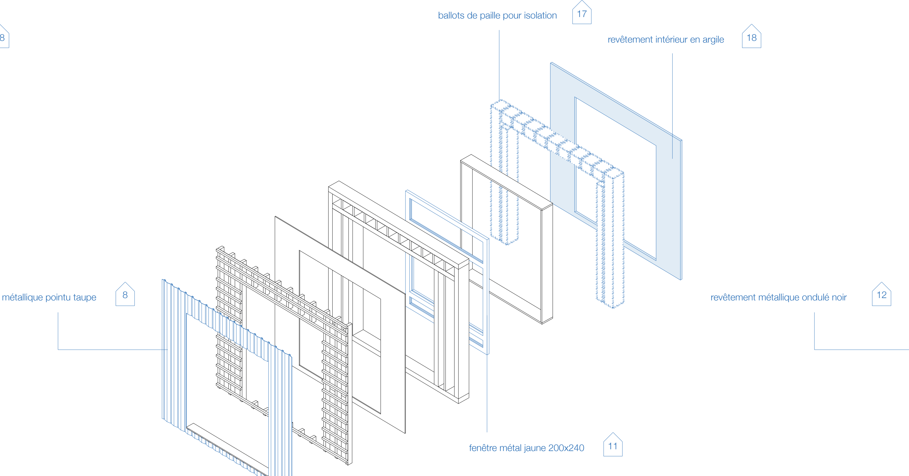
principe de façade échelle 1:50
