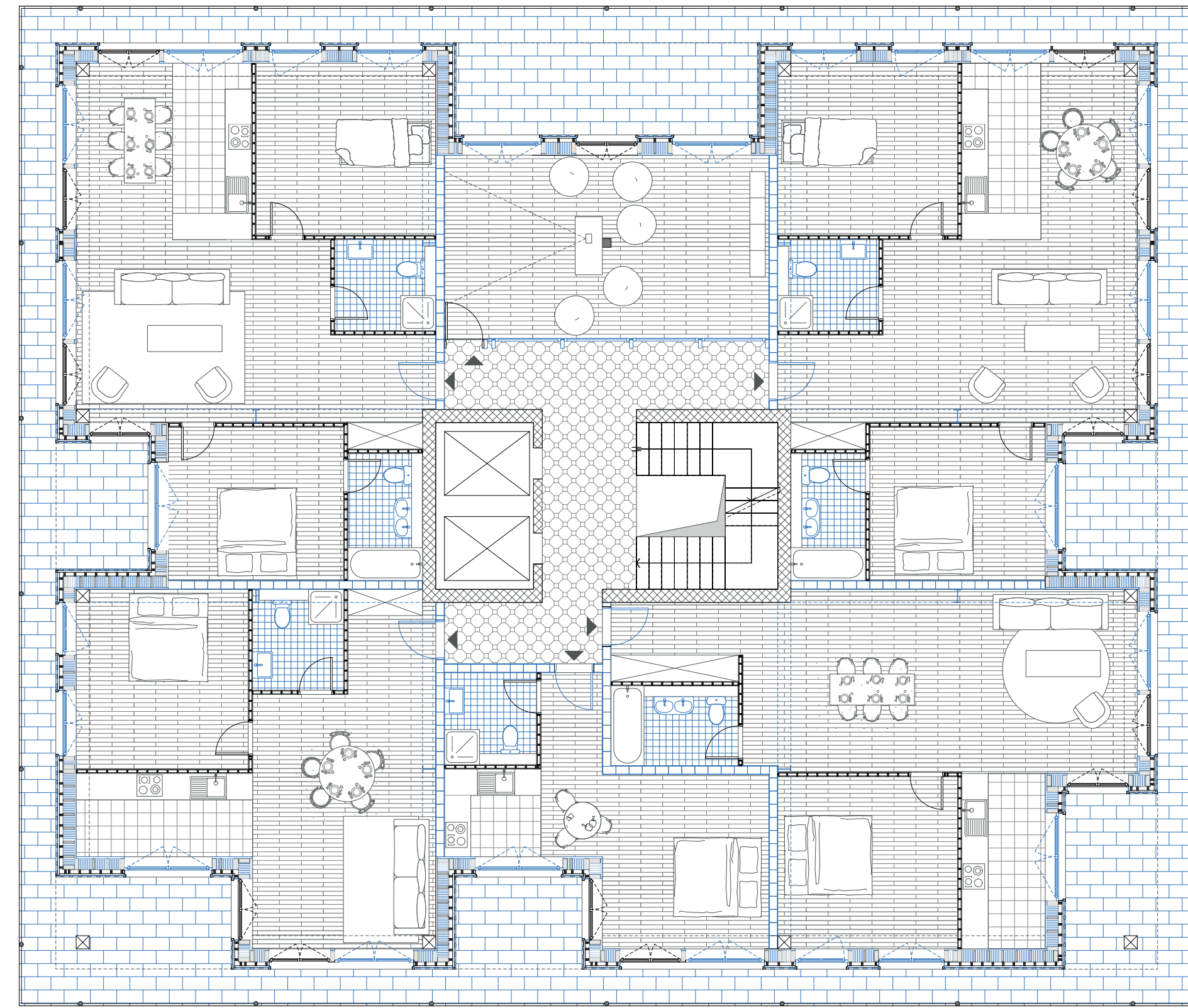
Plan type tour échelle 1:100
