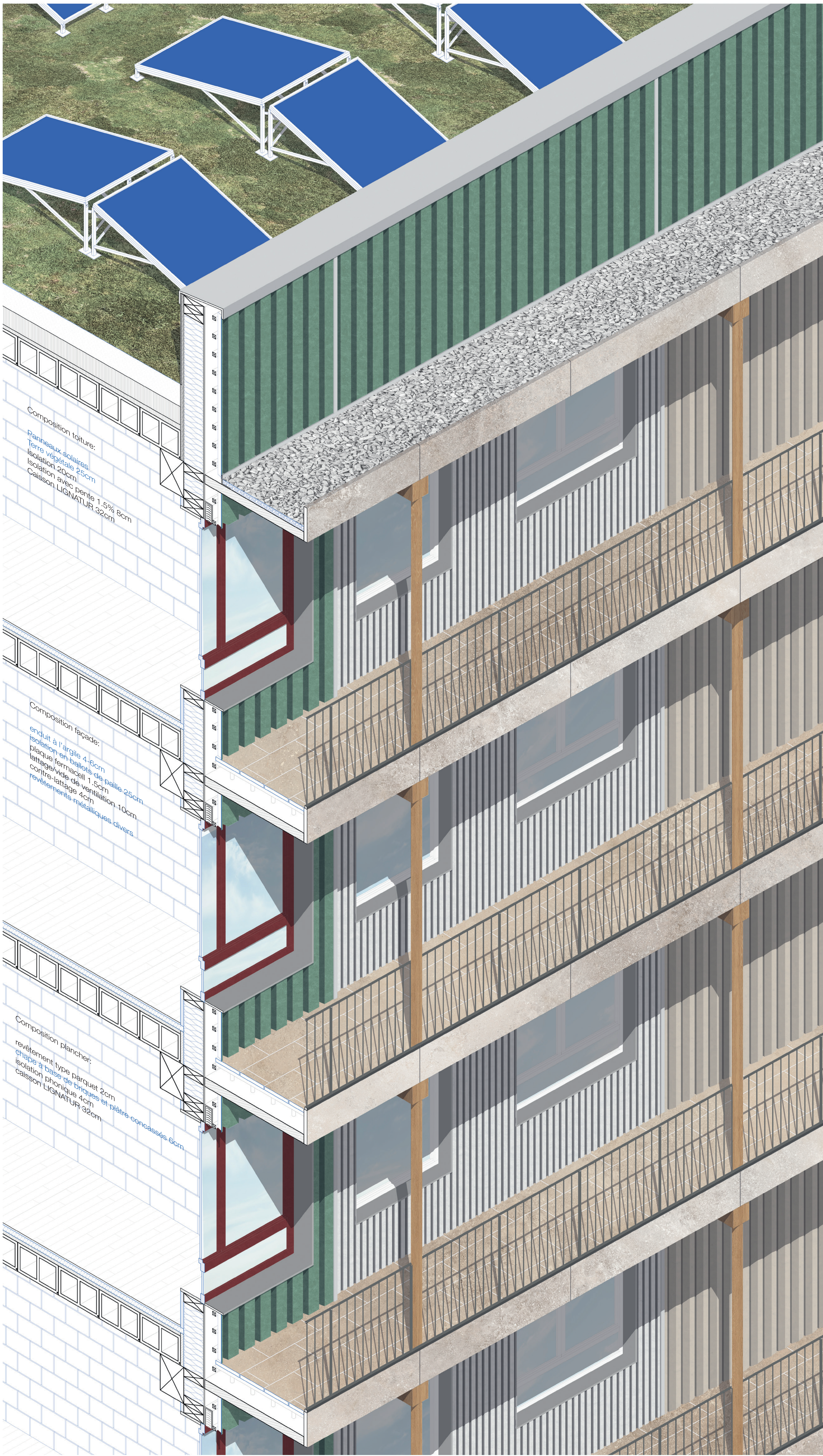
Axonométrie coupée échelle 1:20
