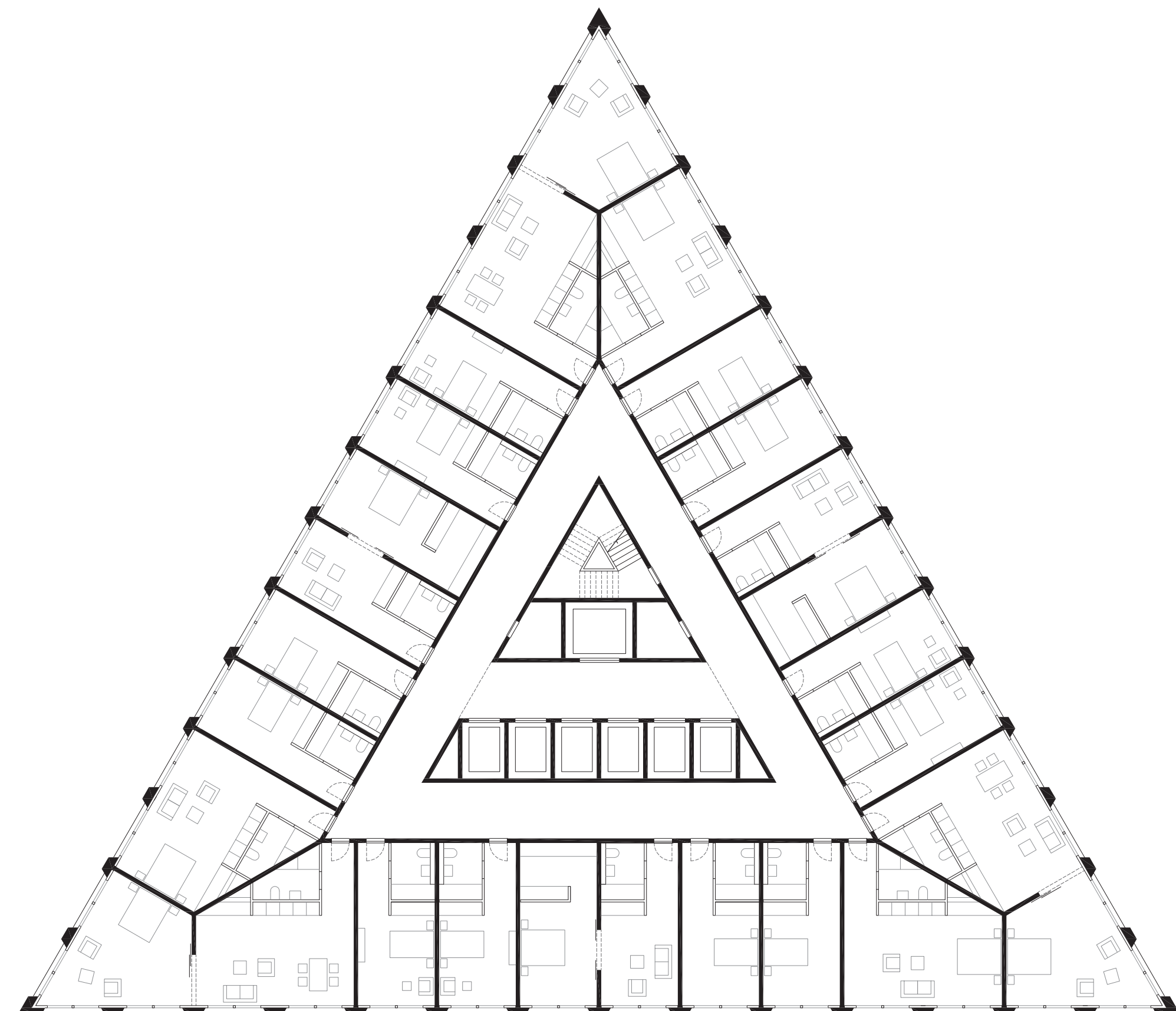
Plan de l'étage type 1/200
