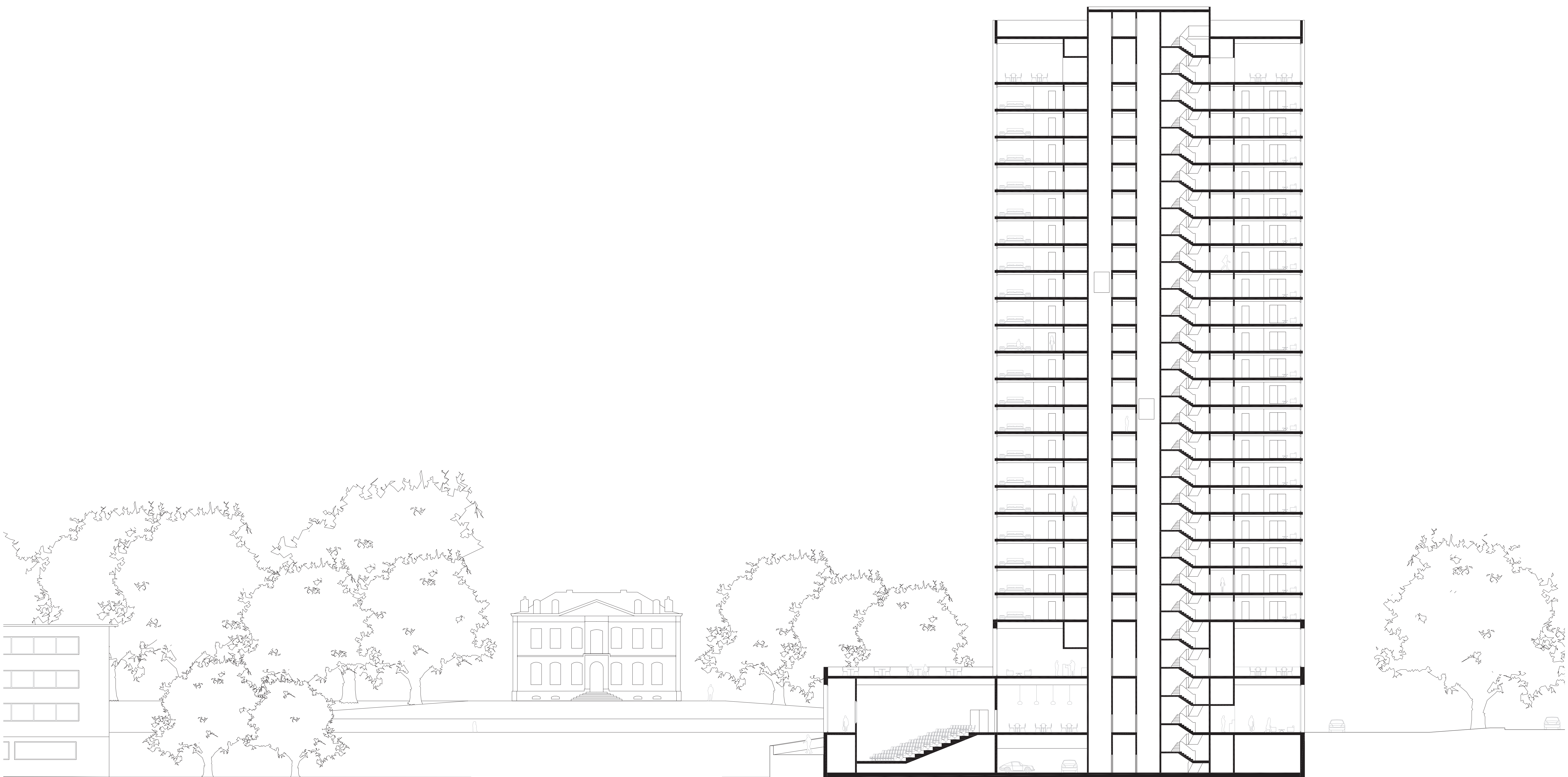
Coupe transversale 1/200
