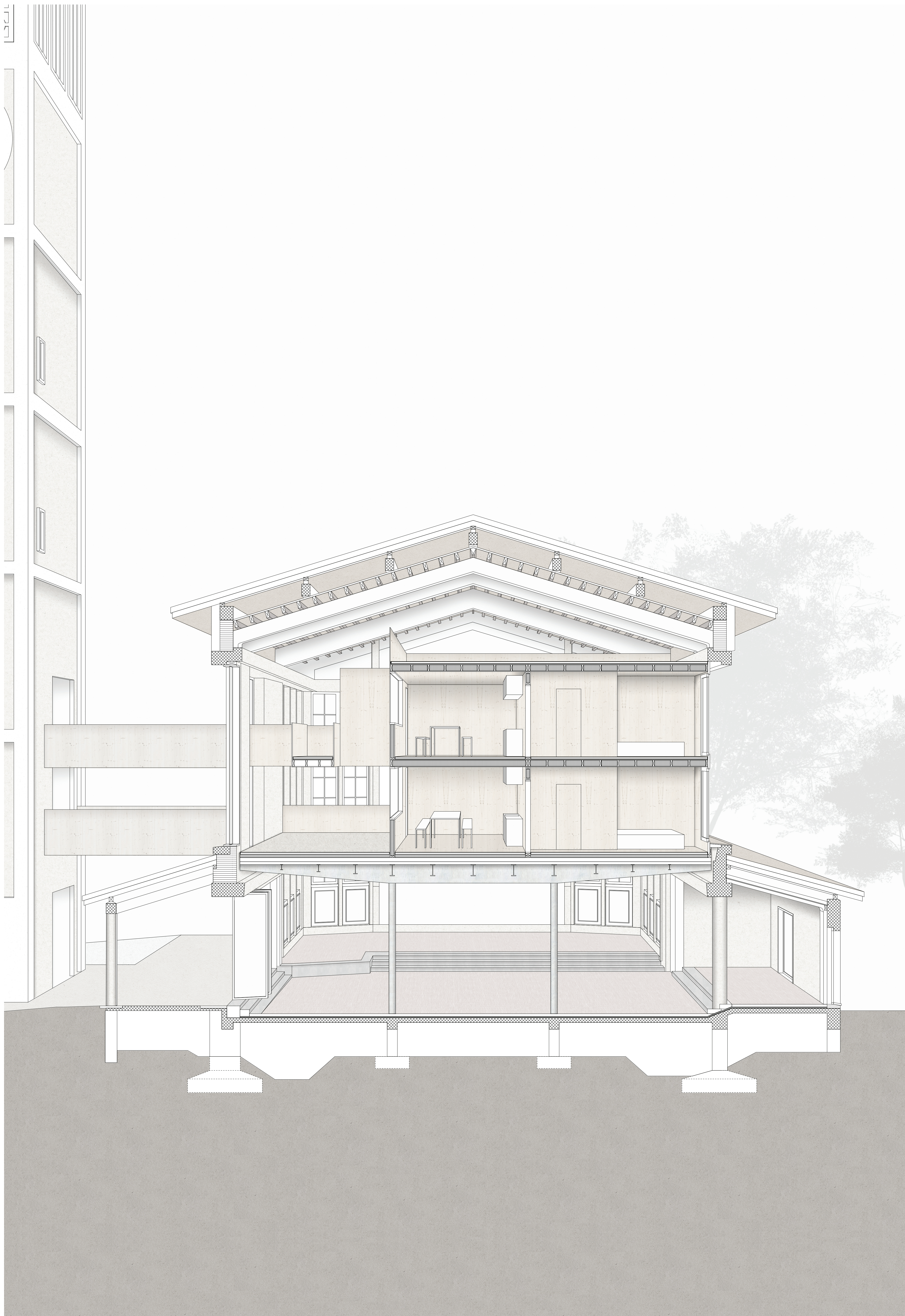
Coupe DD' 1:50
