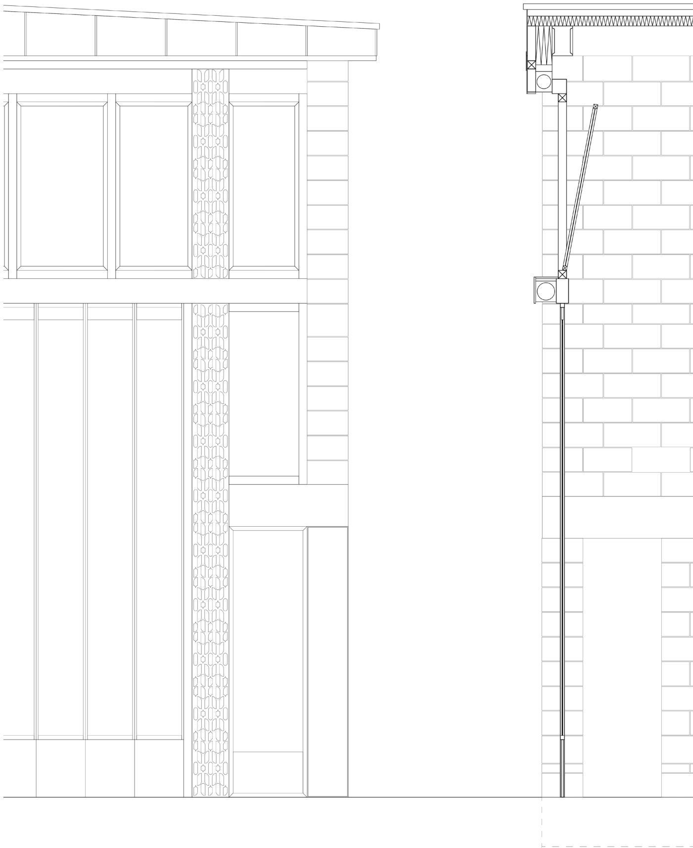
COUPE DE DETAIL : AMPHITHEATRE
