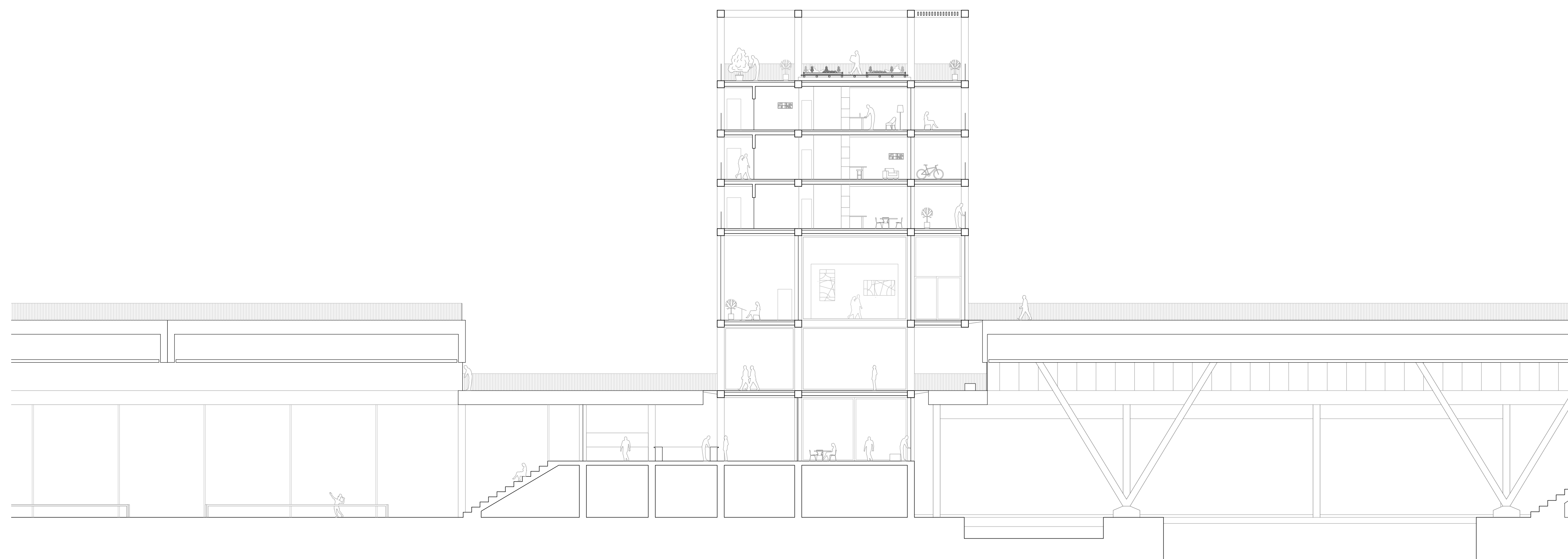
Coupe CC' - 1:200
