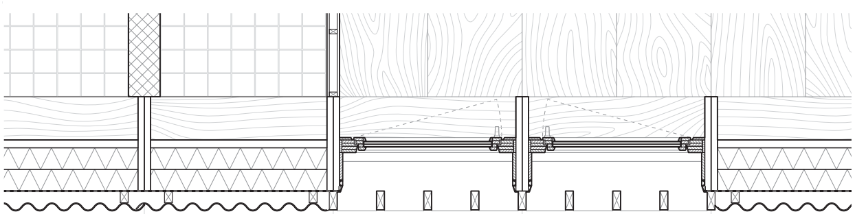
Détail constructif de façade Ateliers
