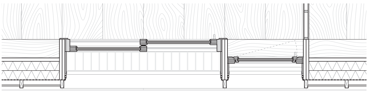
Détail constructif de façade Logements
