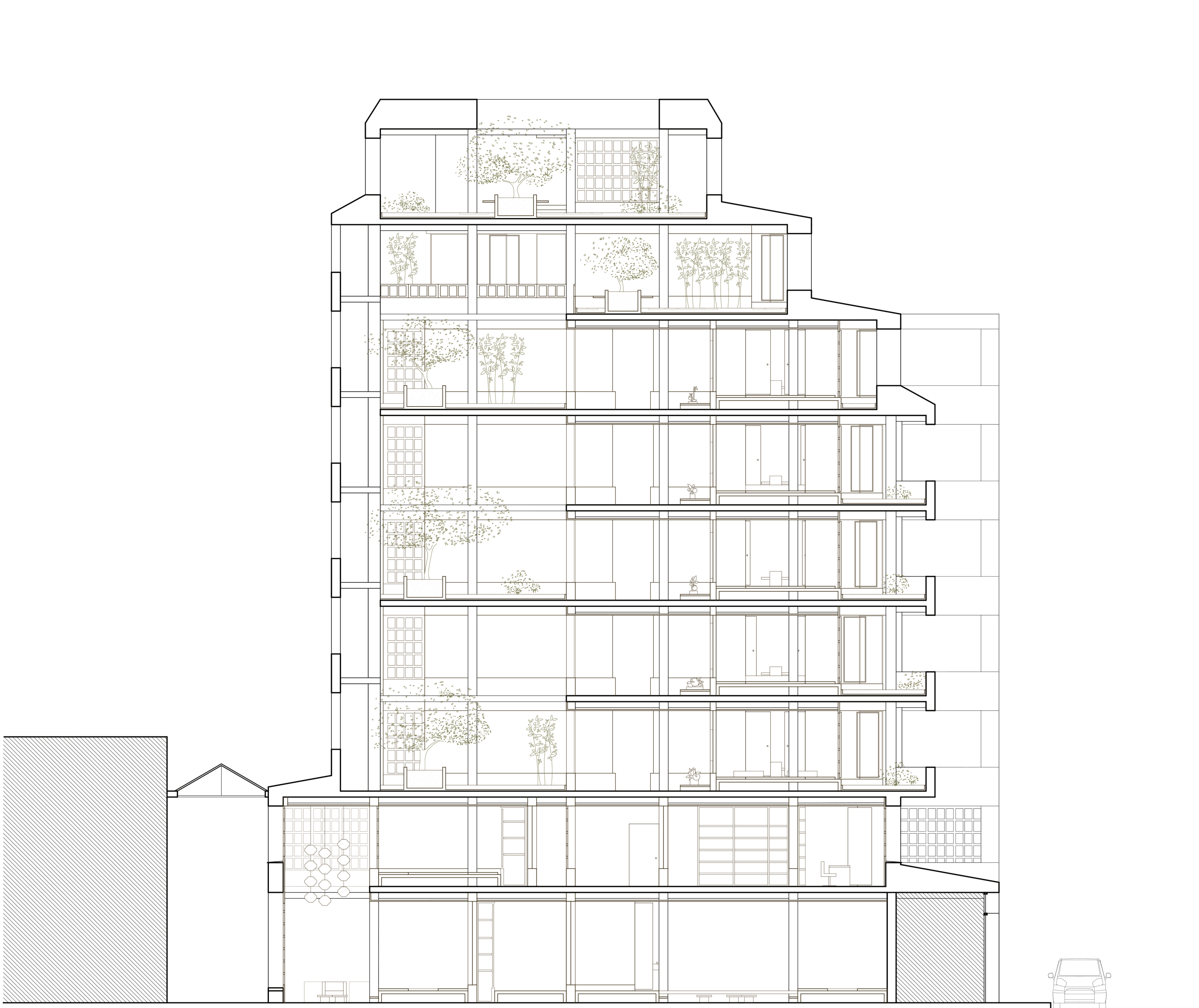
Coupe AA' 1/100e
