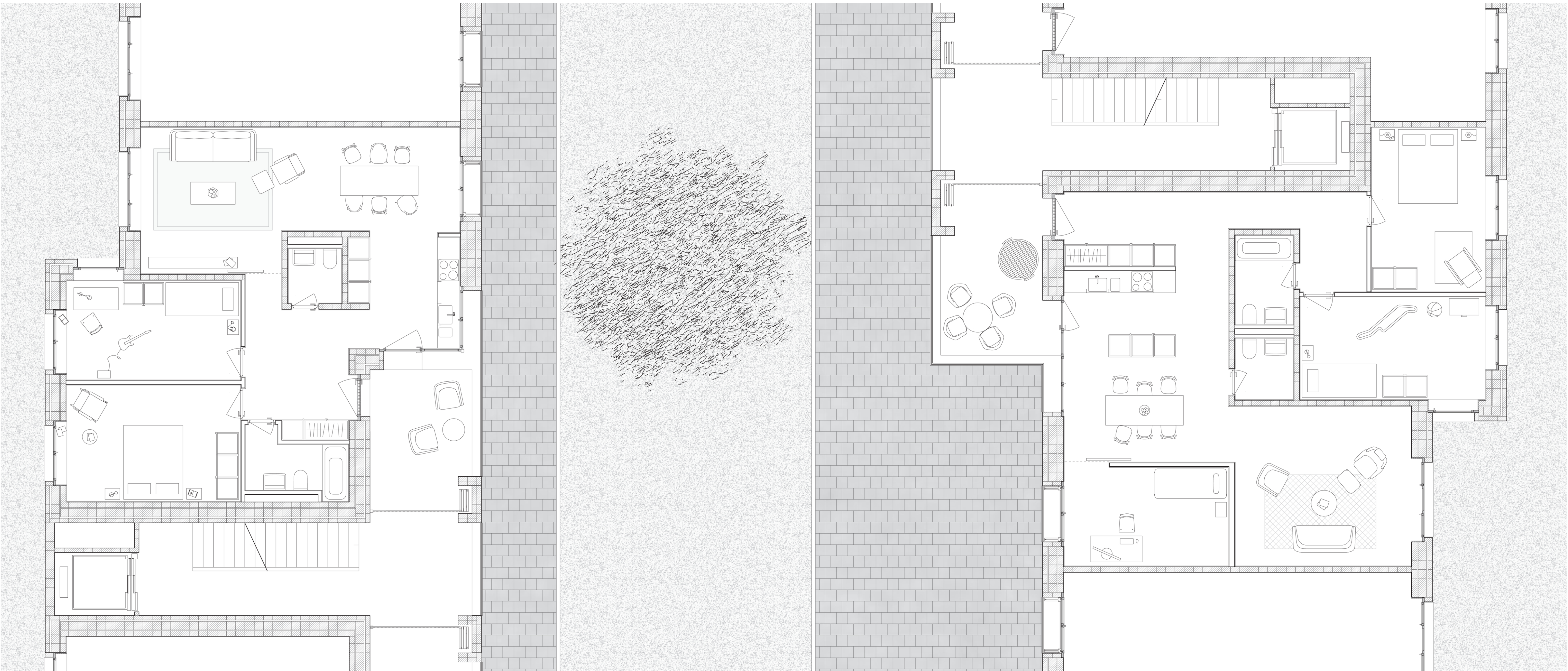
Plan d'appartements types sur la nouvelle rue, 1:50
