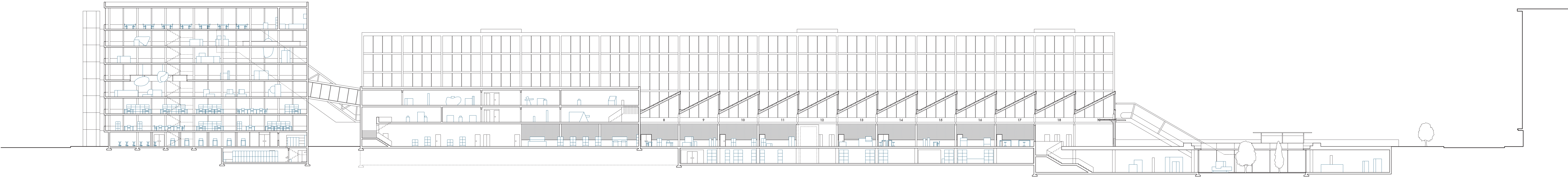
coupe longitudinale, 1:250
