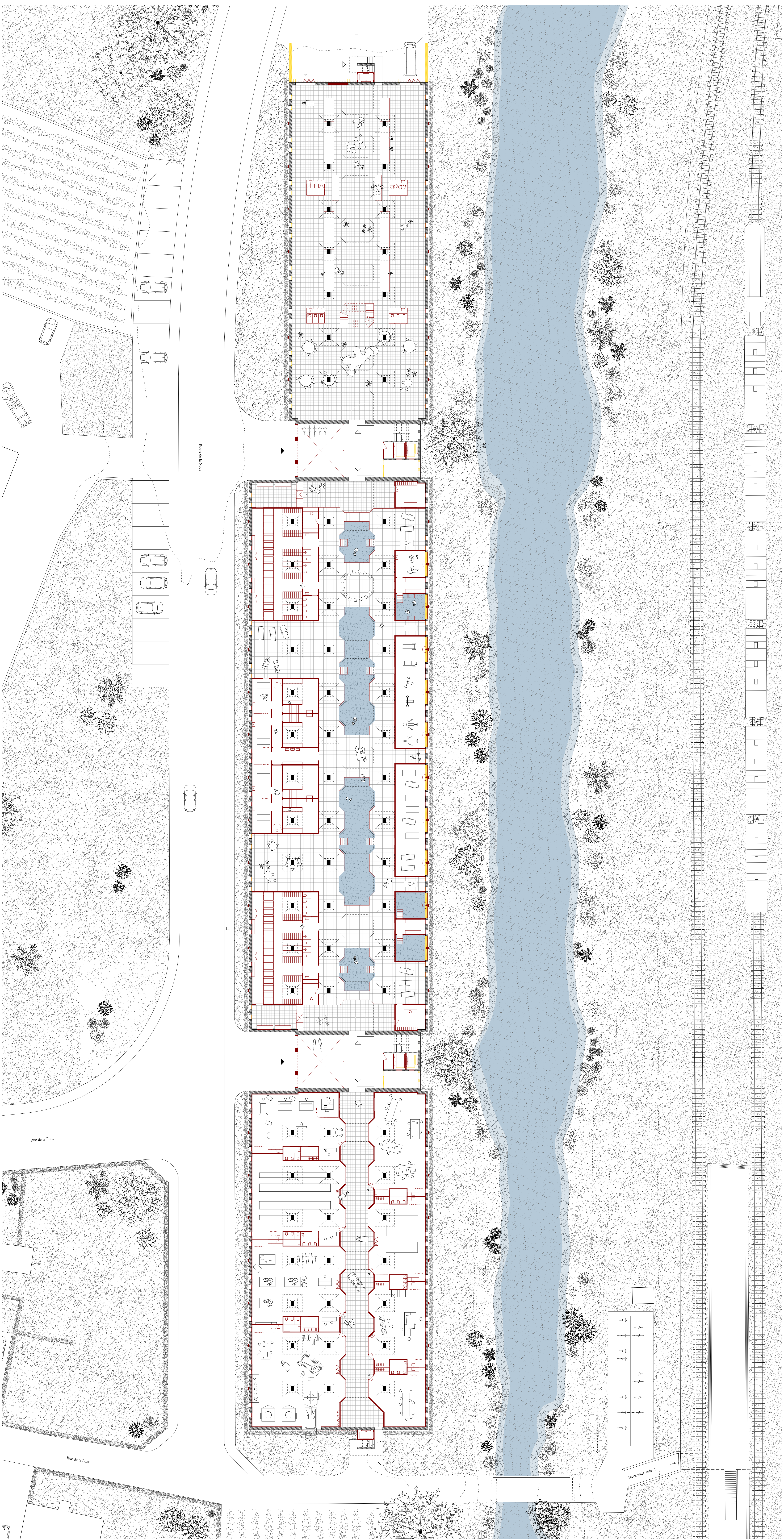
PLAN REZ-DE-CHAUSSEE 1:200
