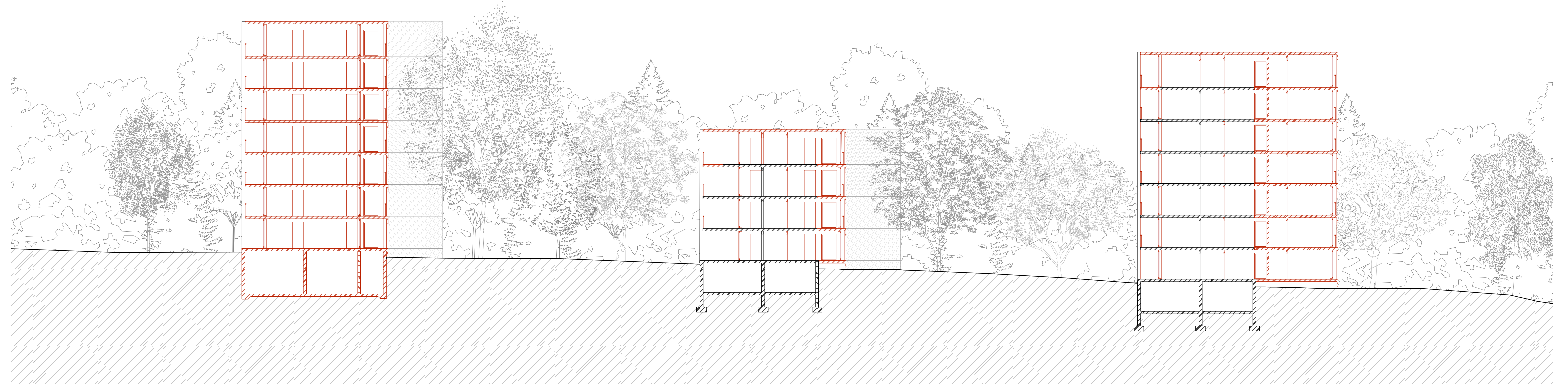
COUPE B-B SUR LES DIFFÉRENTS TYPES D'AJOUT 1:200
