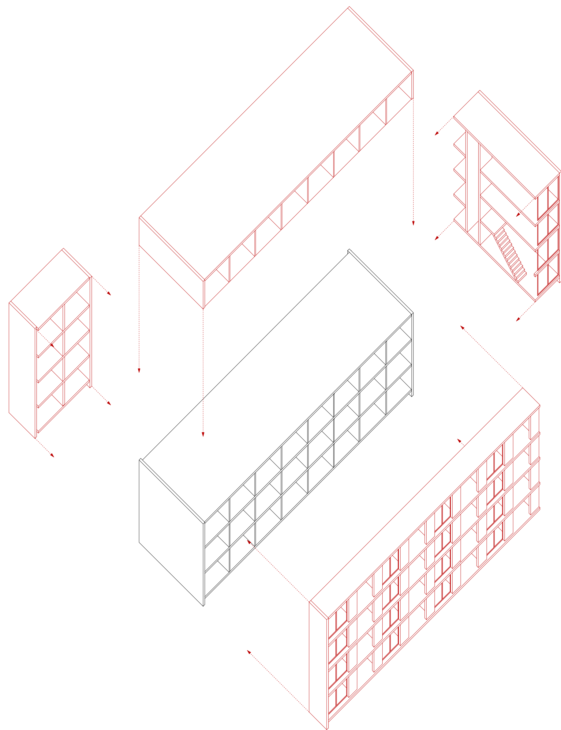
AXONOMETRIE DES DIFFÉRENTS TYPES D'AJOUT
