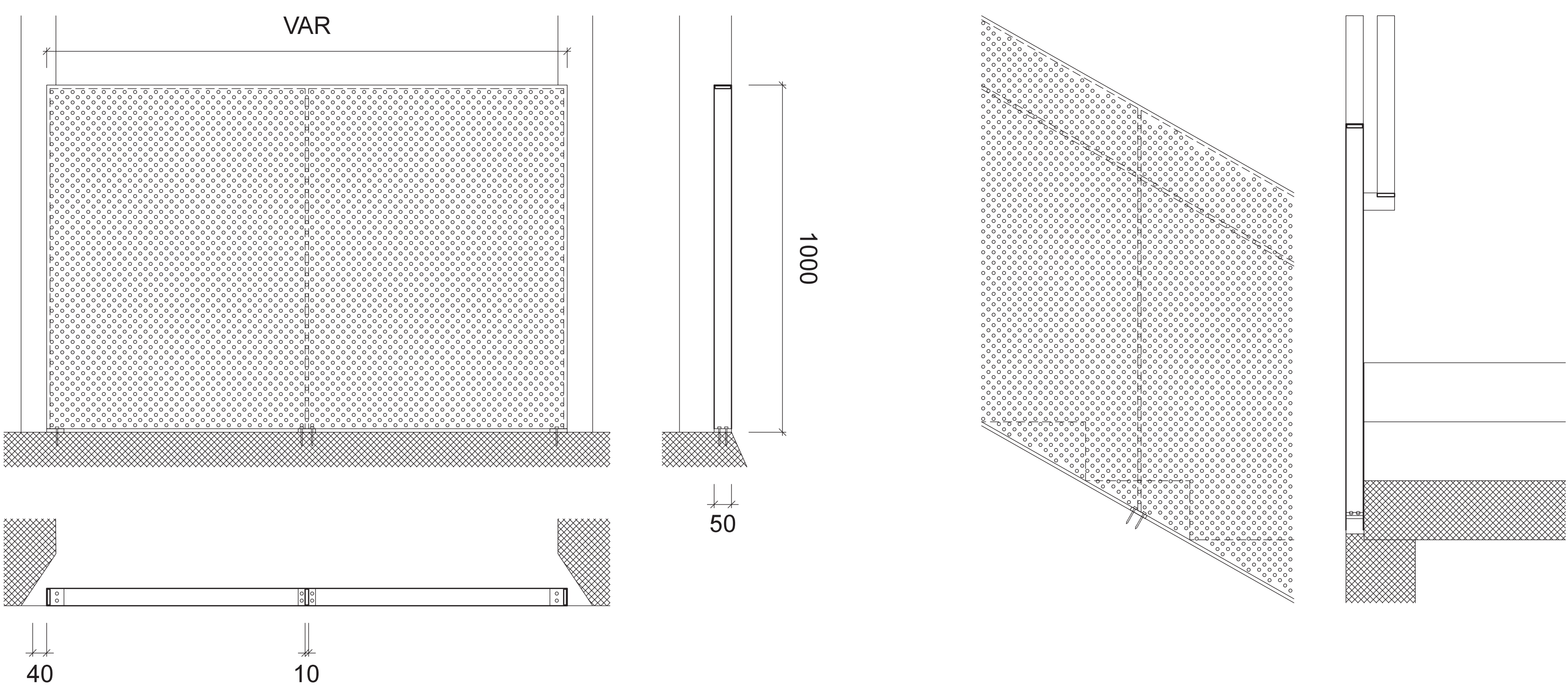
DÉTAIL DES GARDE-CORPS _ 1:10
