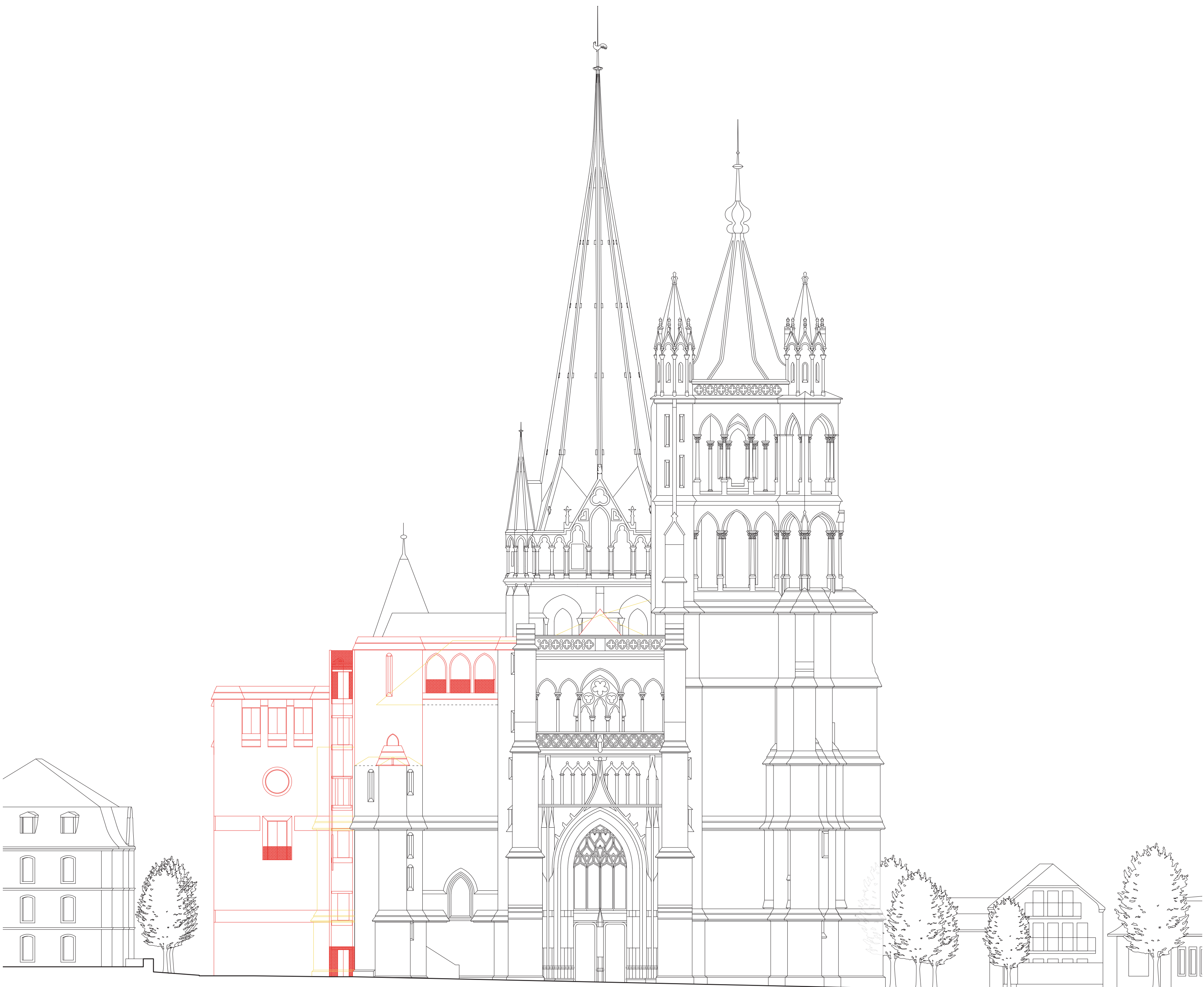
ÉLEVATION OUEST _ 1:200
