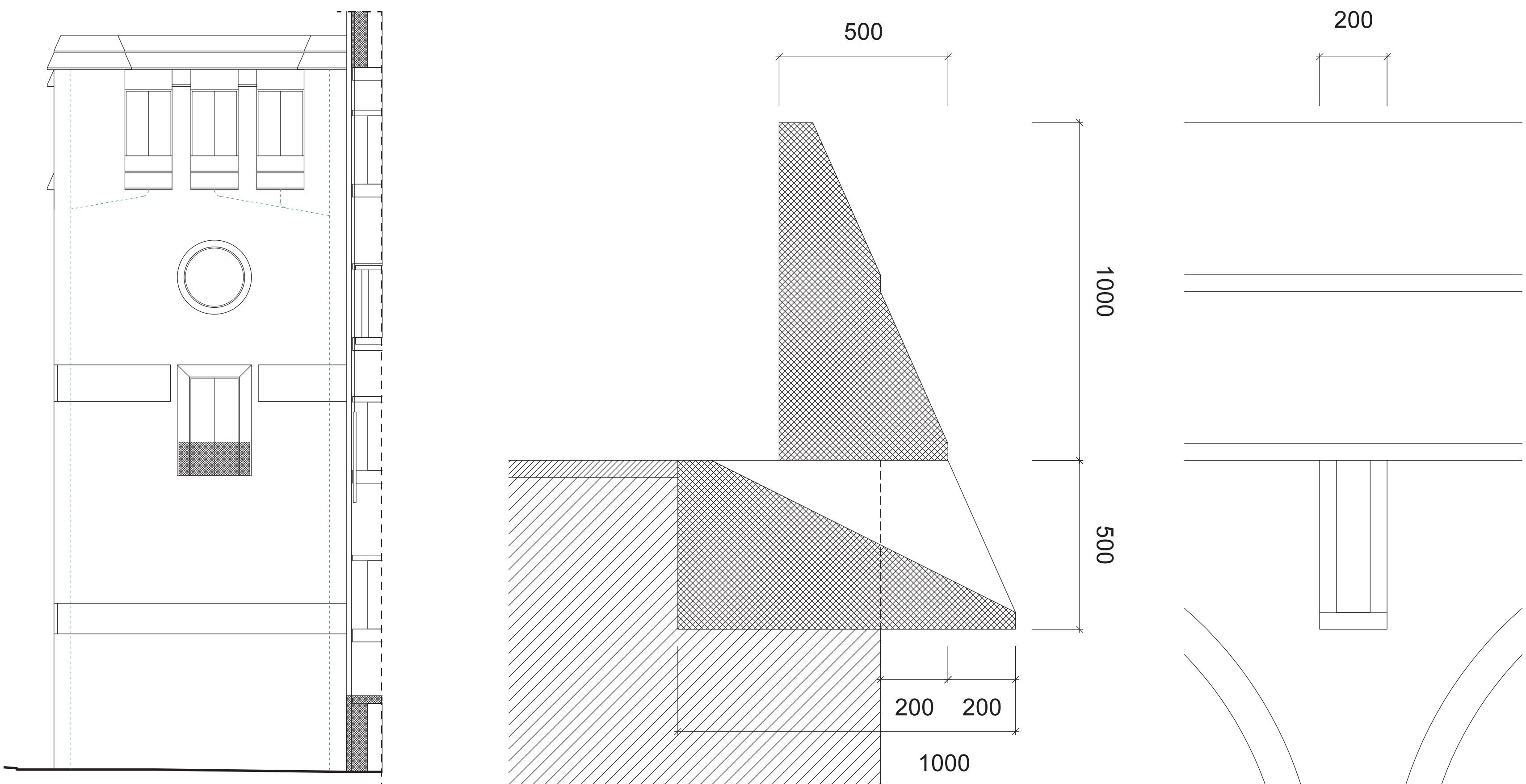
DESCENTE DES EAUX DU BÂTIMENT NEUF _ 1:200
