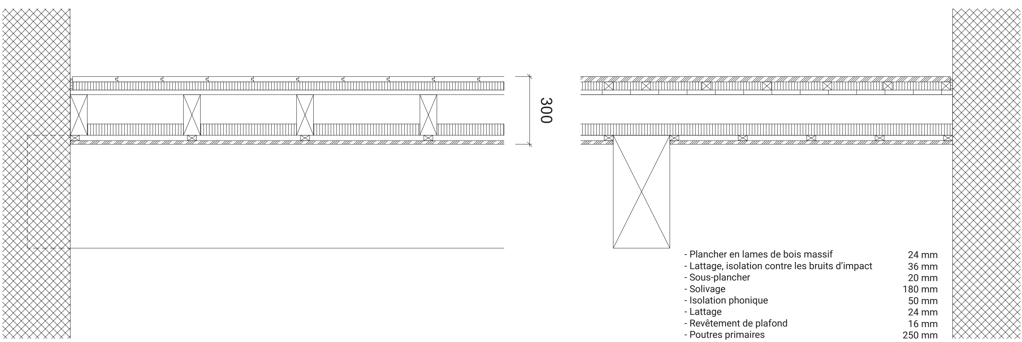
DÉTAIL DES PLANCHERS DU BÂTIMENT NEUF _ 1:10
