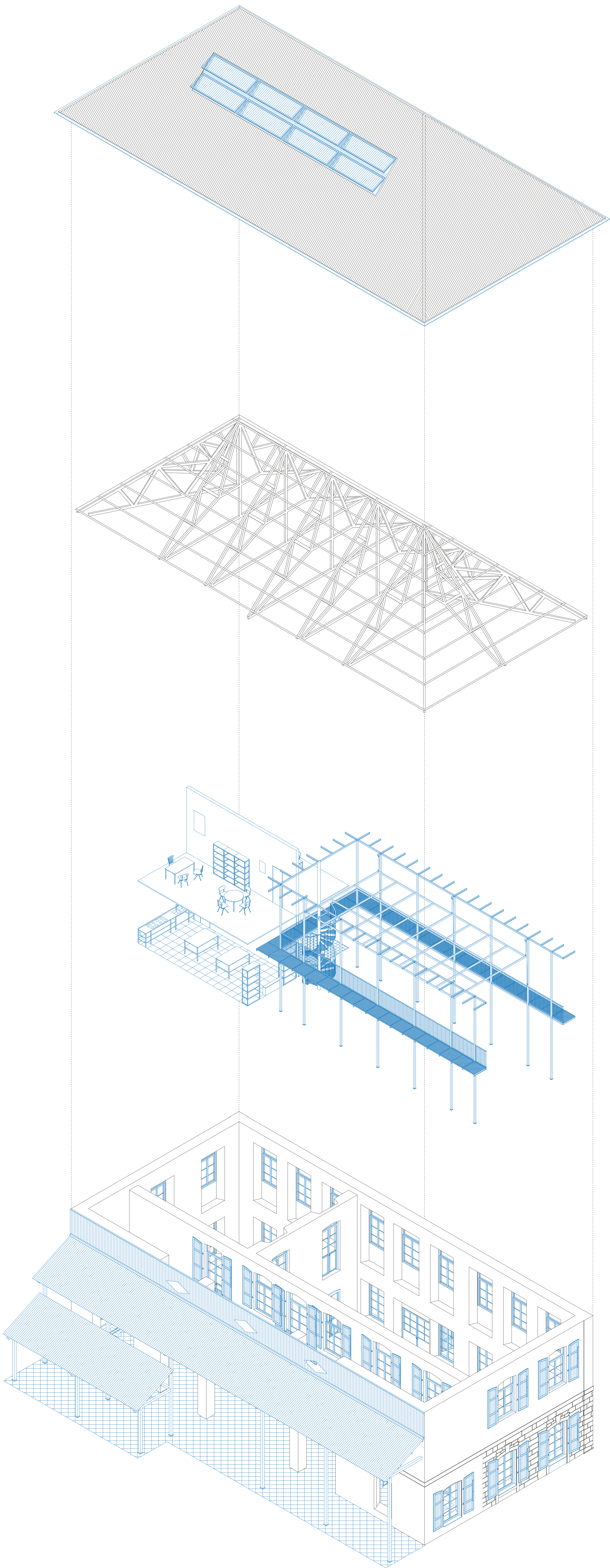
AXONOMETRIE
