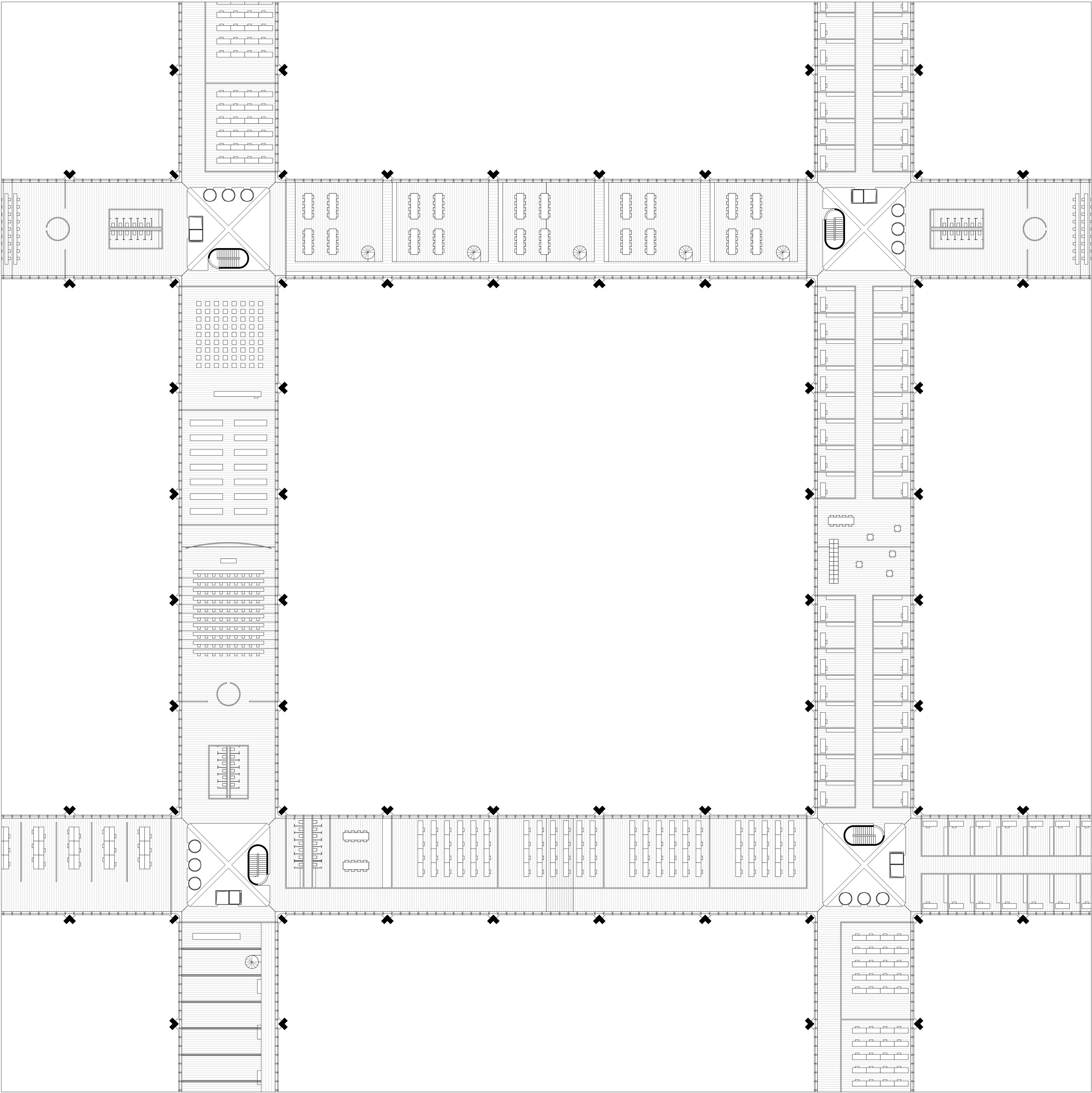
Niveau 1-3 - Ecole - 1:200
