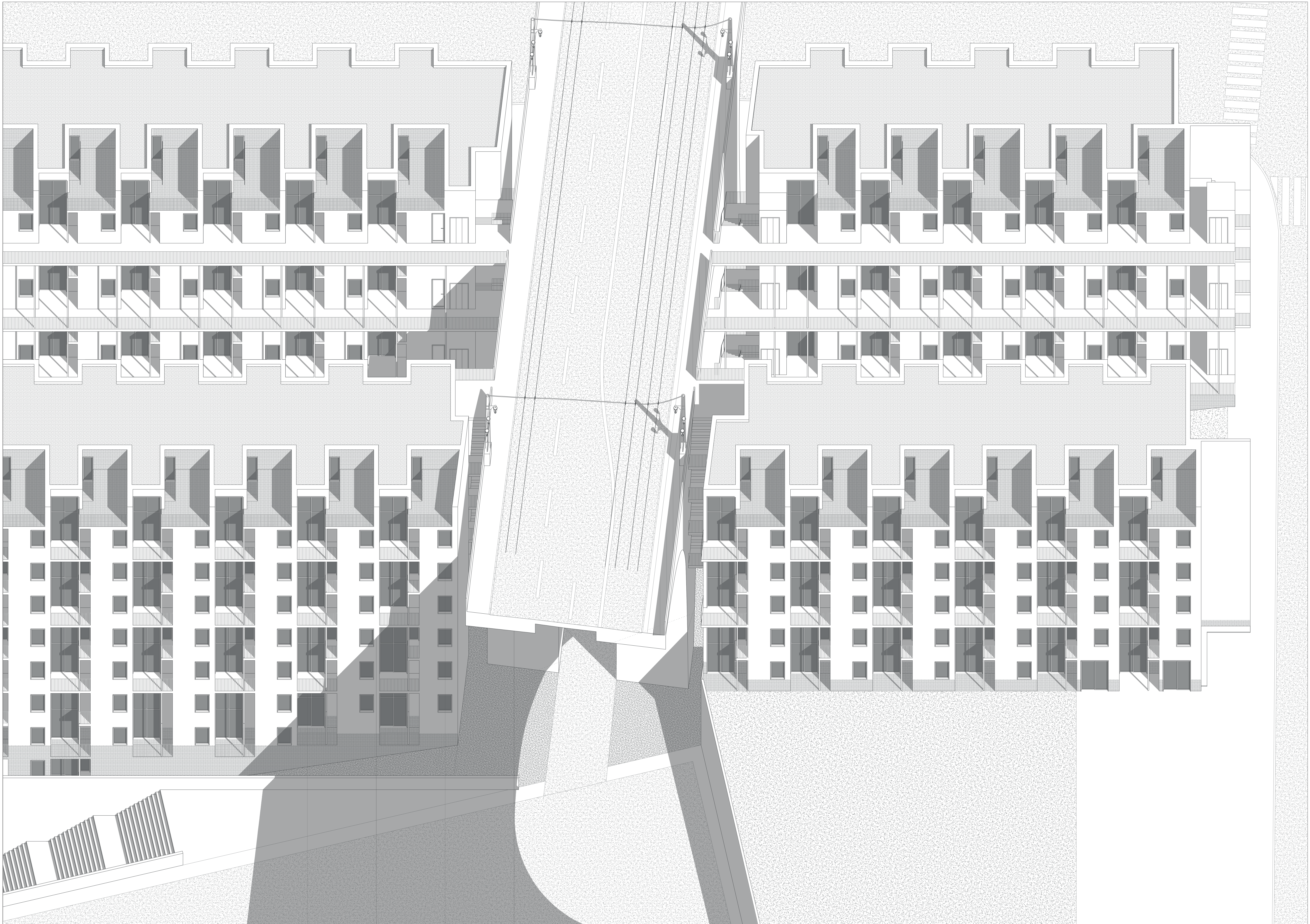
Axonométrie frontale partielle 1:100
