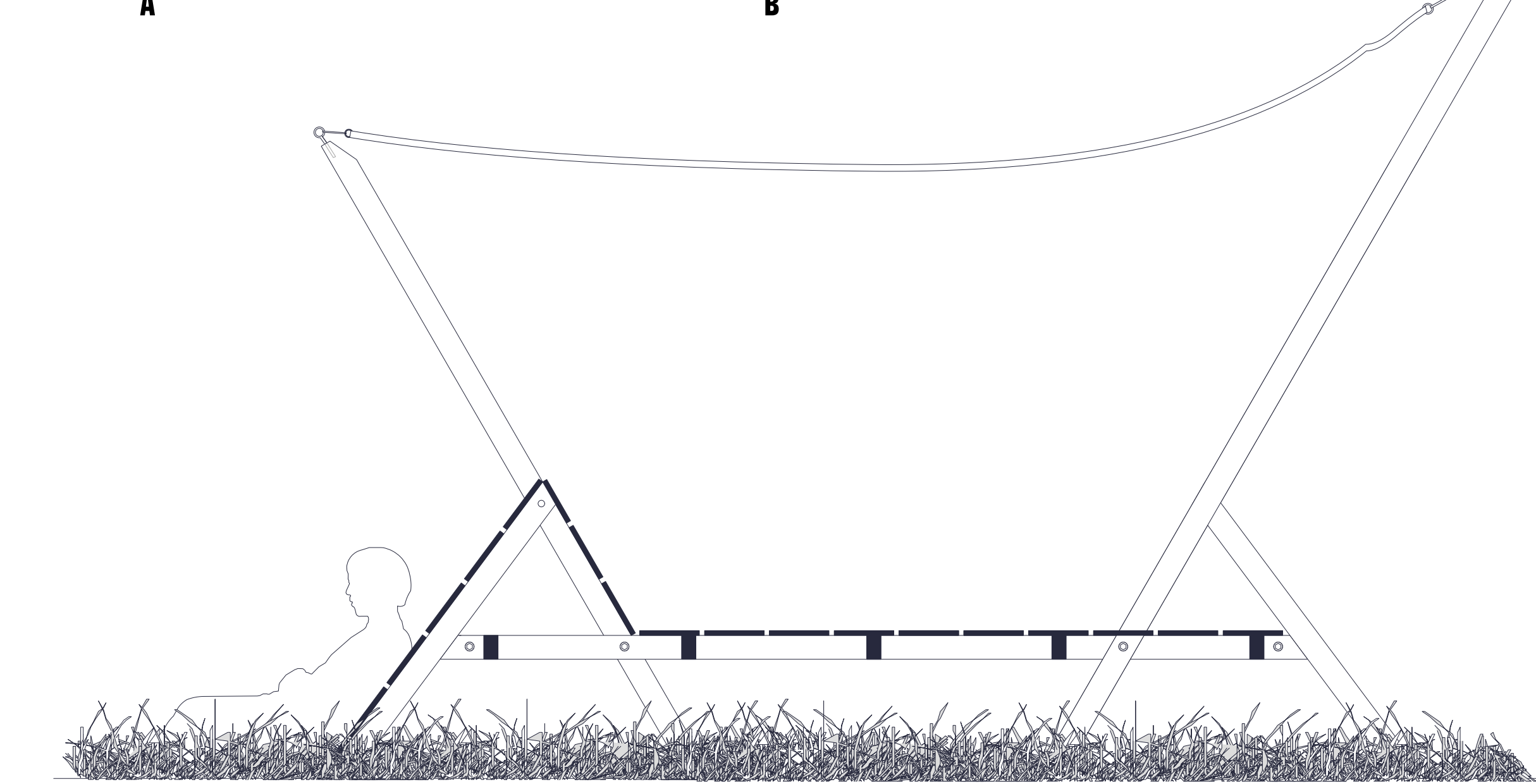
ASSISES "VOILE" COUPE B 1:20
