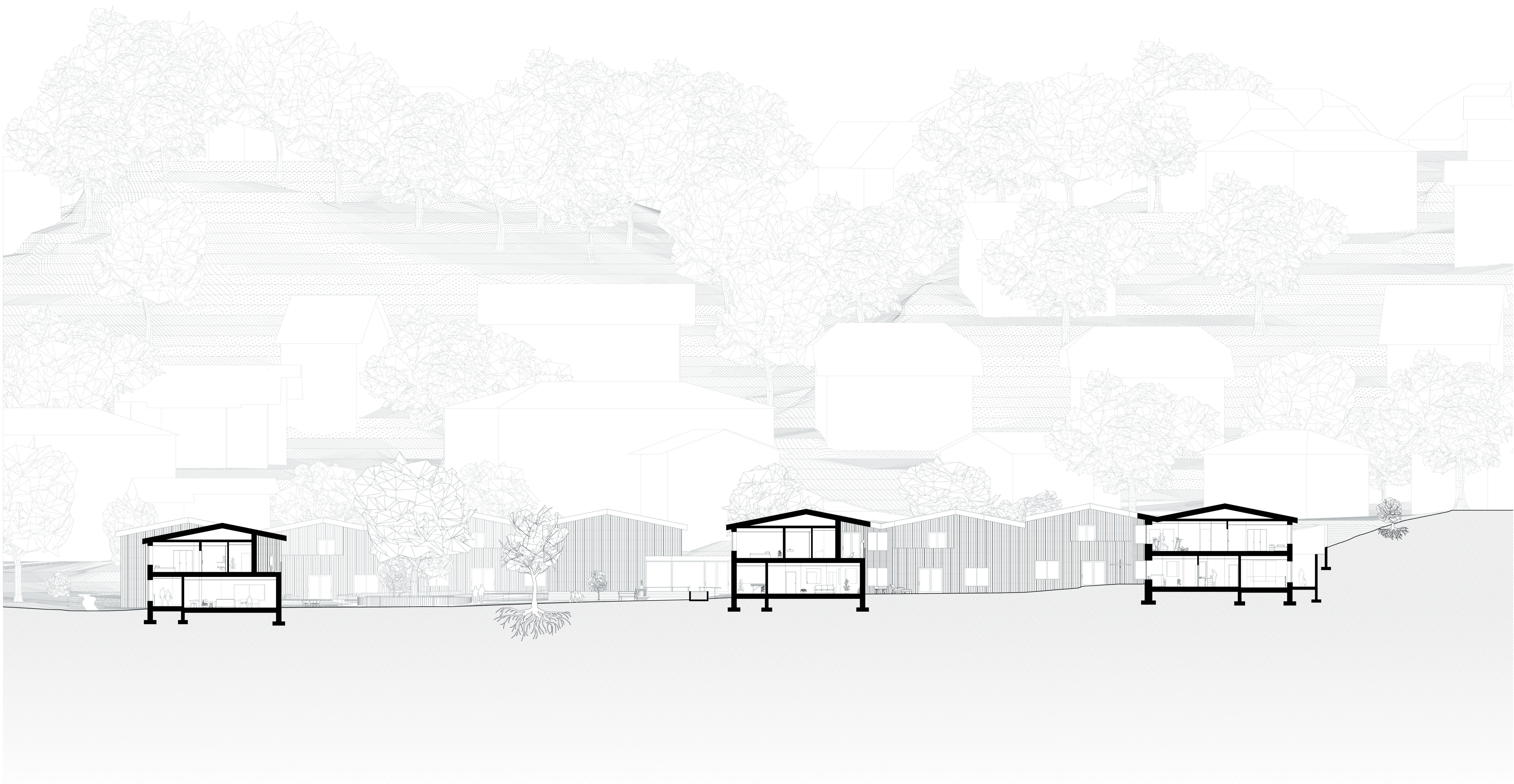
Coupe AA 1:200
