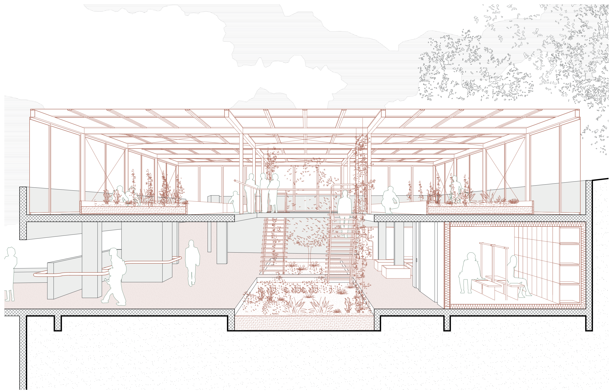
Coupe perspective - Serres expérimentales - Echelle 1/50
