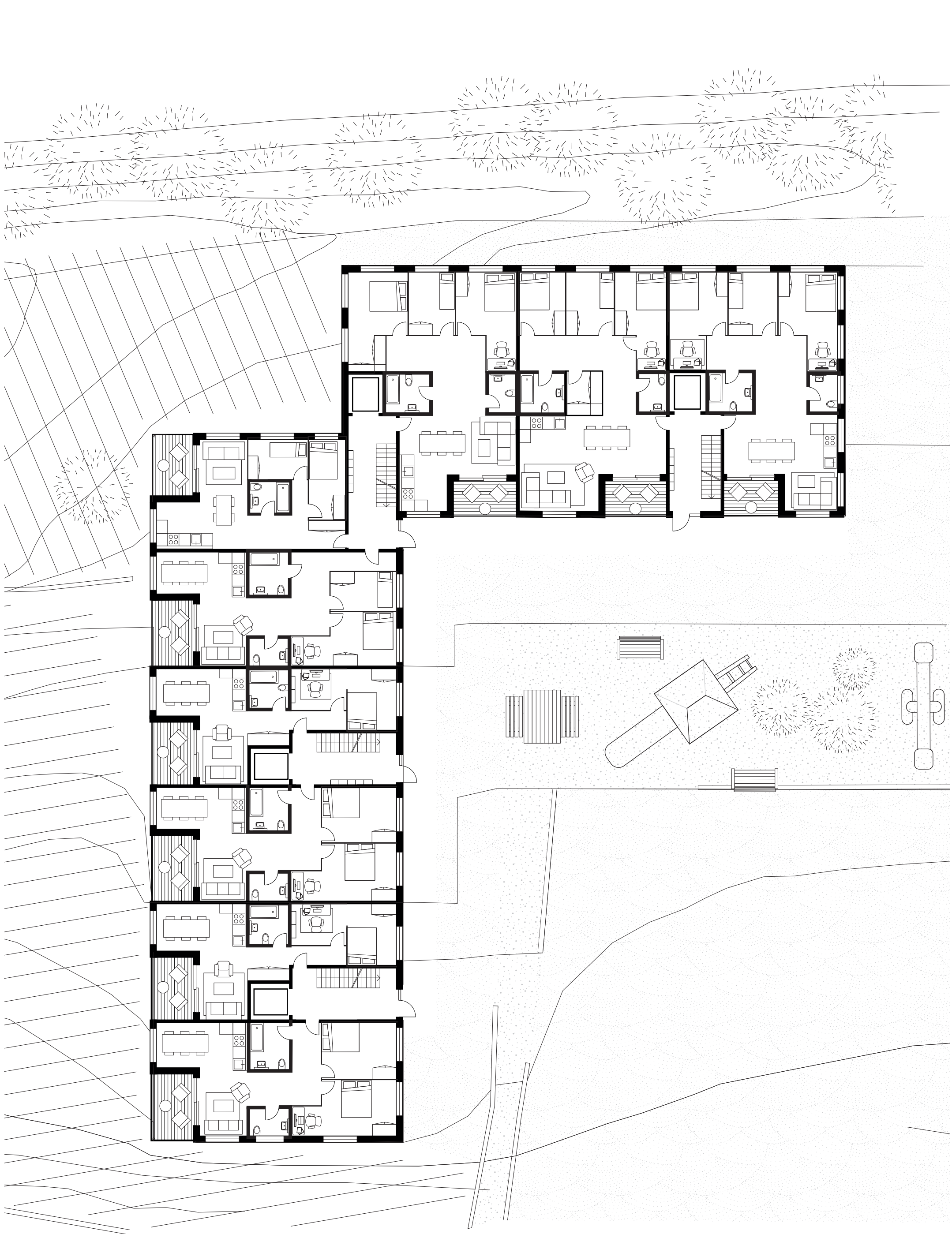
Plan des étages significatifs 1:200
