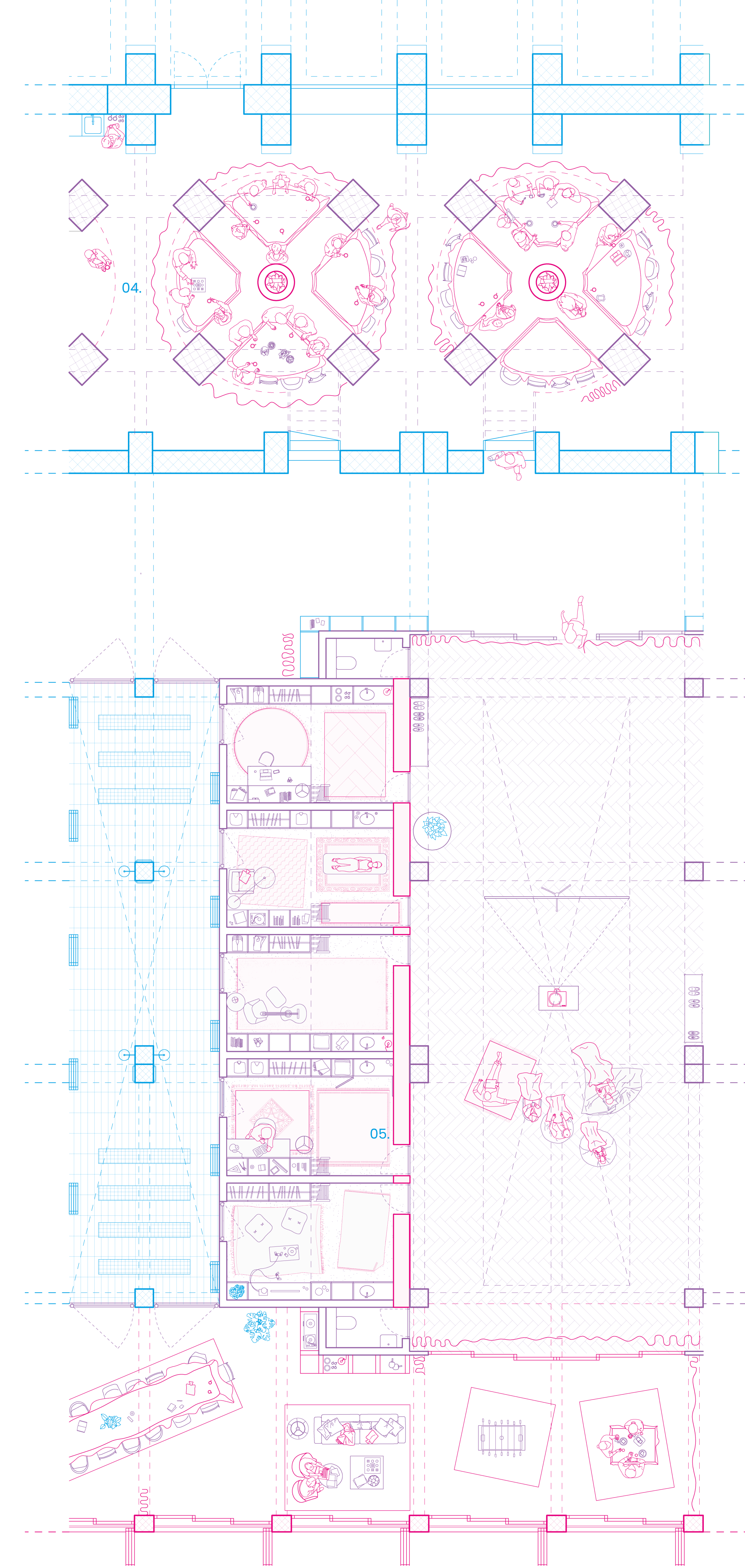
plan usages hivernaux - R+1 1:66
