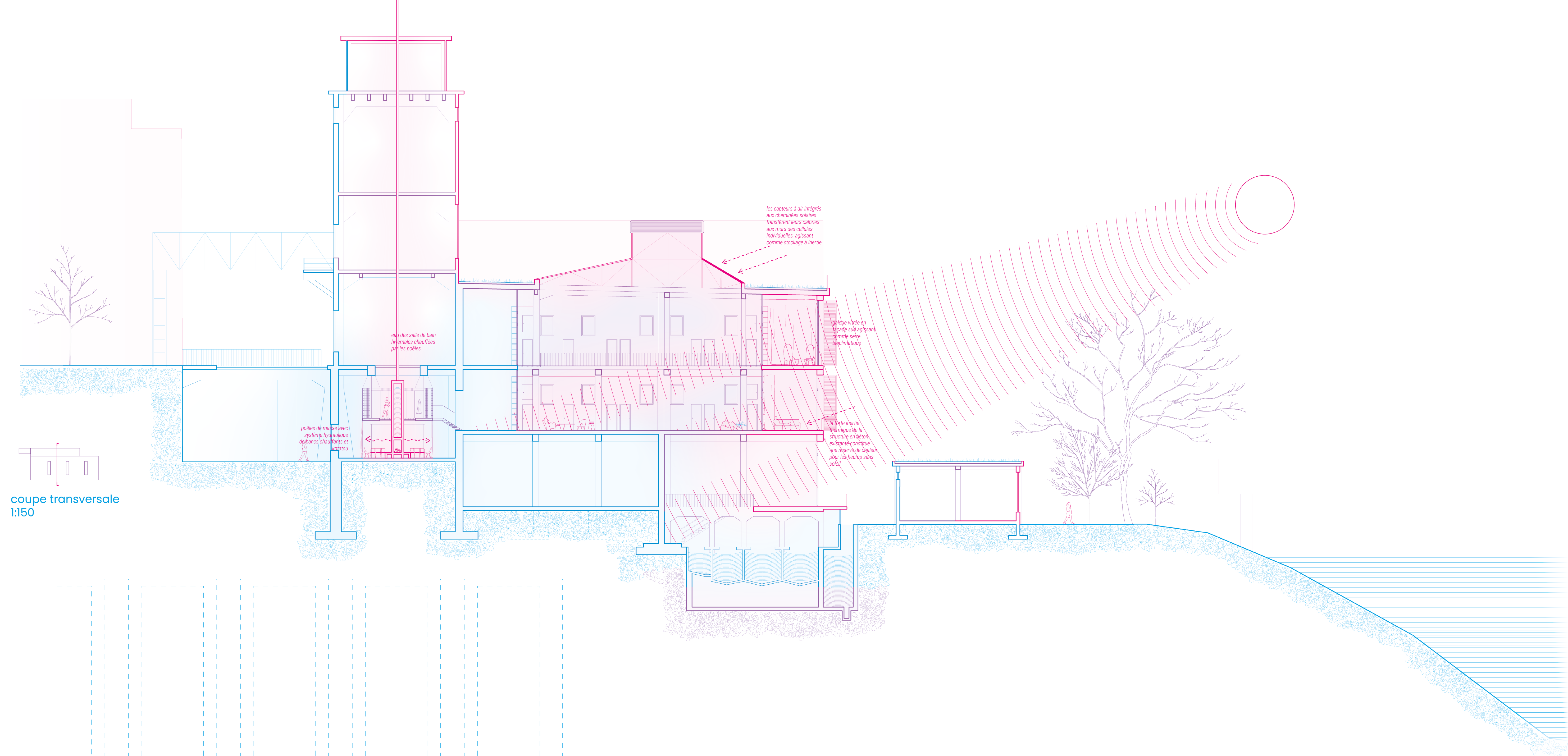
coupe longitudinale et élévation sud 1:150
