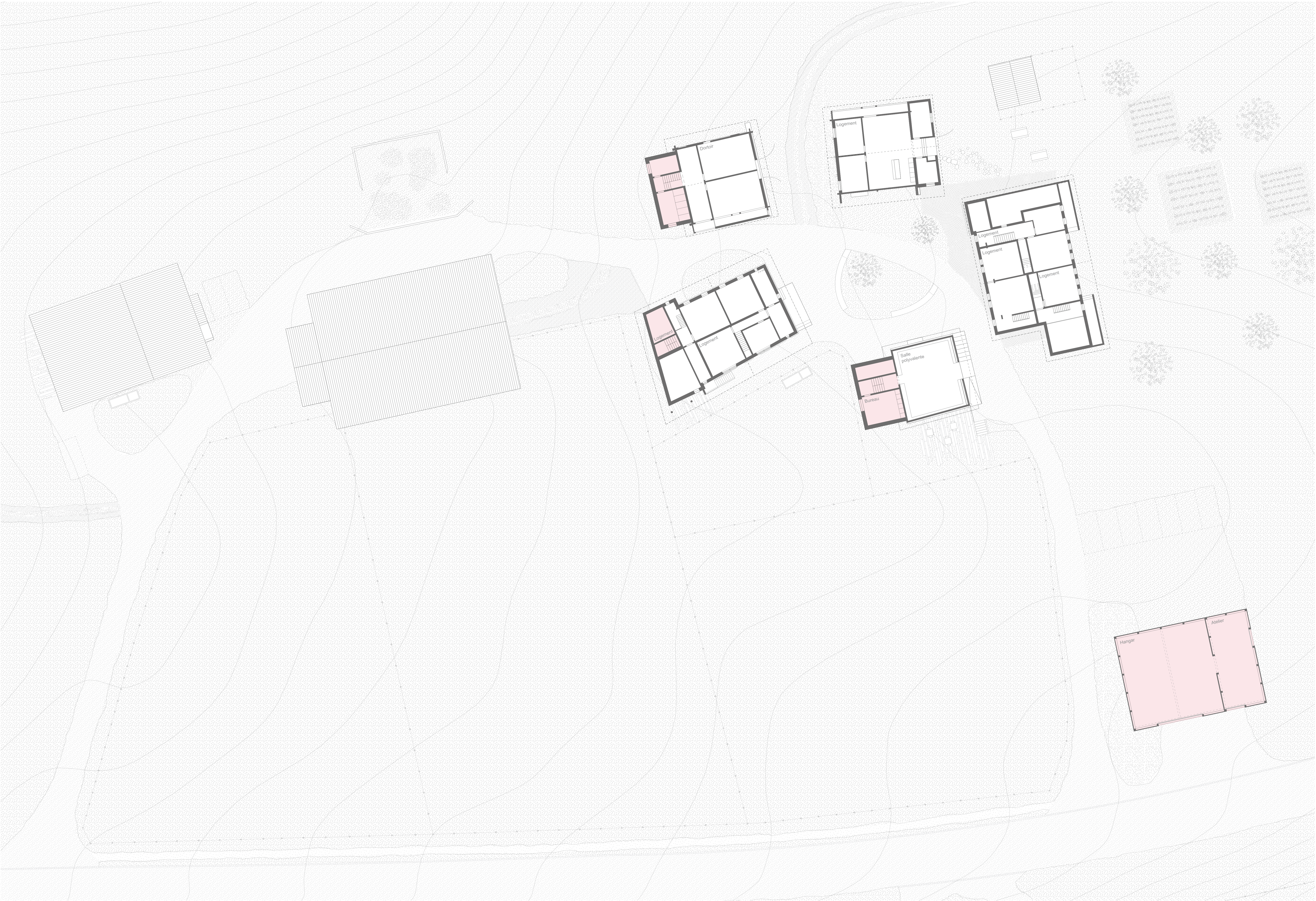
Plan niveau hangar, 1:200
