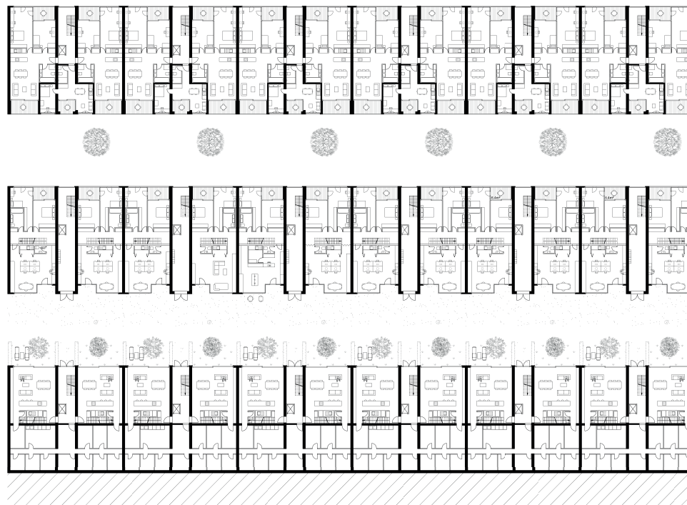
PLANS APPARTEMENTS BATIMENT COTE FRONT URBAIN 1:200, DE BAS EN HAUT: REZ INFERIEUR, REZ SUPERIEUR, ETAGE TYPE
