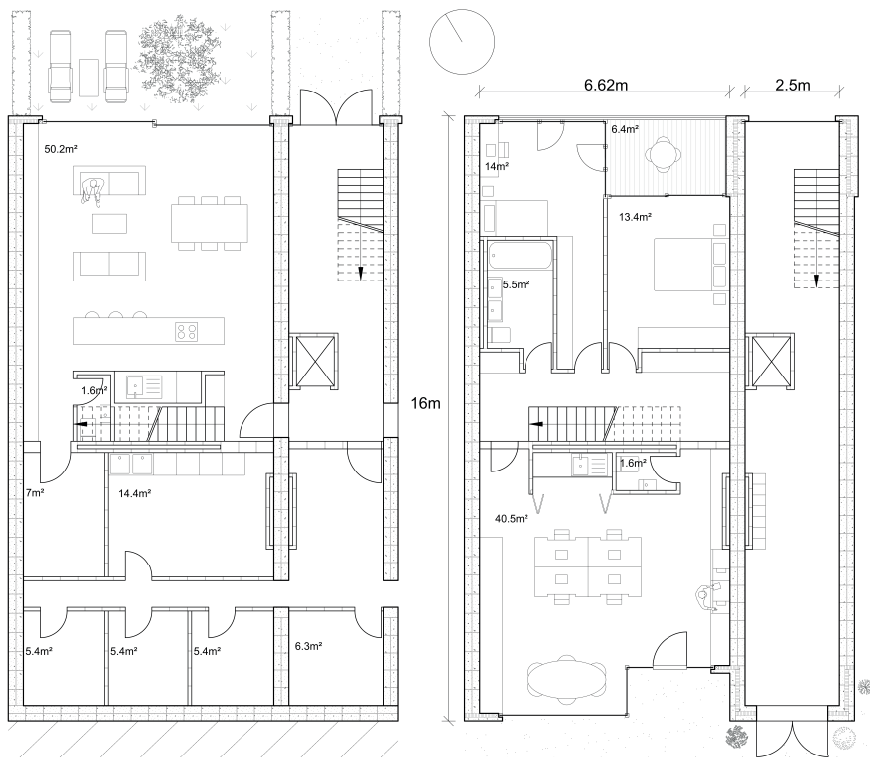
PLAN APPARTEMENTS BATIMENT COTE FRONT URBAIN 1:50, HAUT: ETAGE TYPE, BAS GAUCHE: REZ INFERIEUR, BAS DROITE: REZ SUPERIEUR
