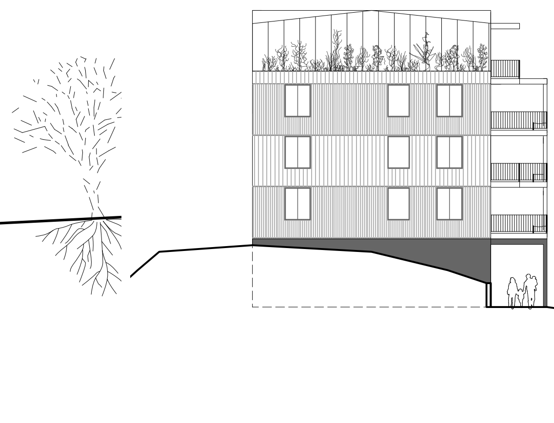
Élévation ouest: 1:200
