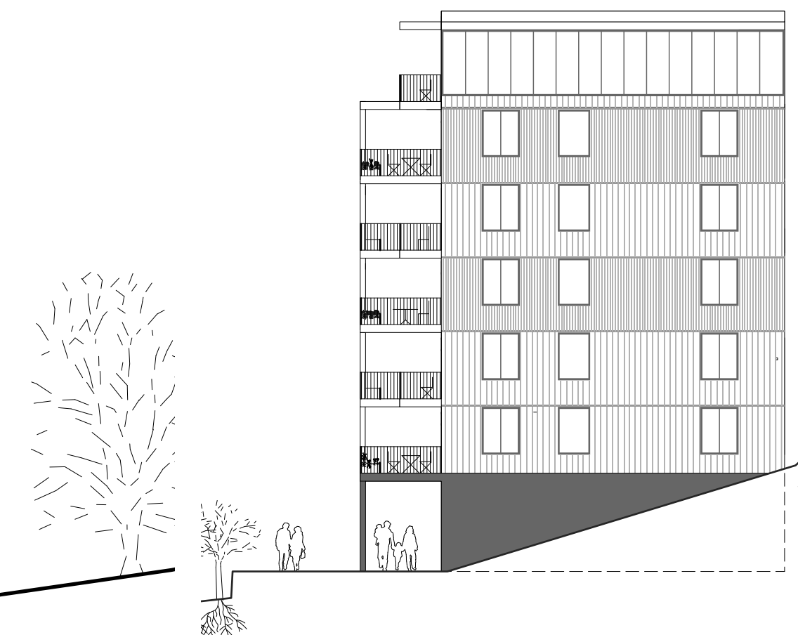
Élévation ouest: 1:200
