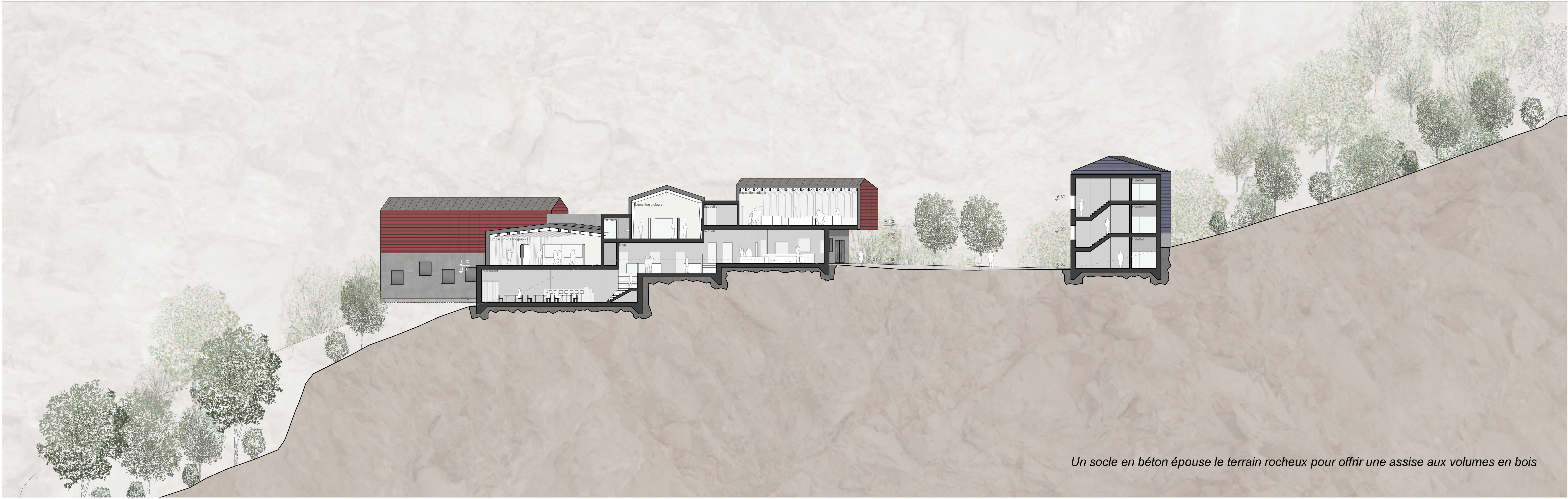
Coupe EE 1:200
