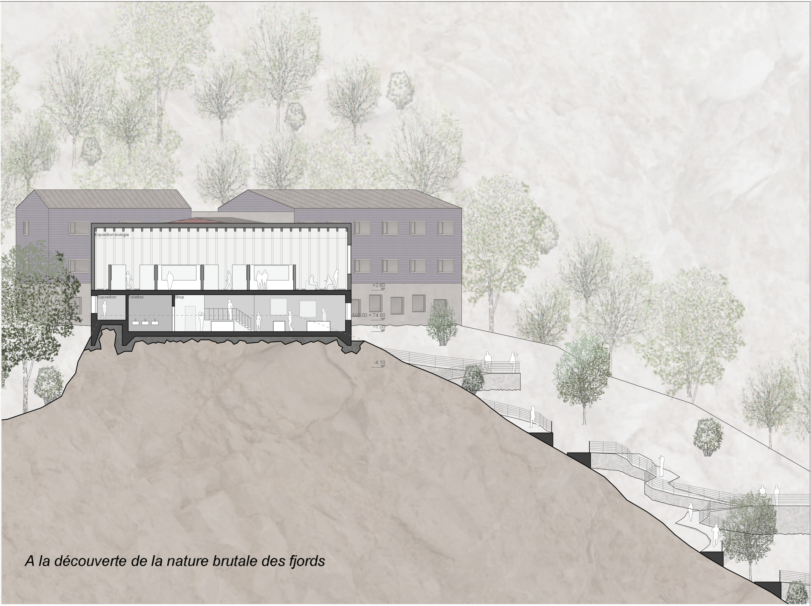
Coupe FF 1:200
