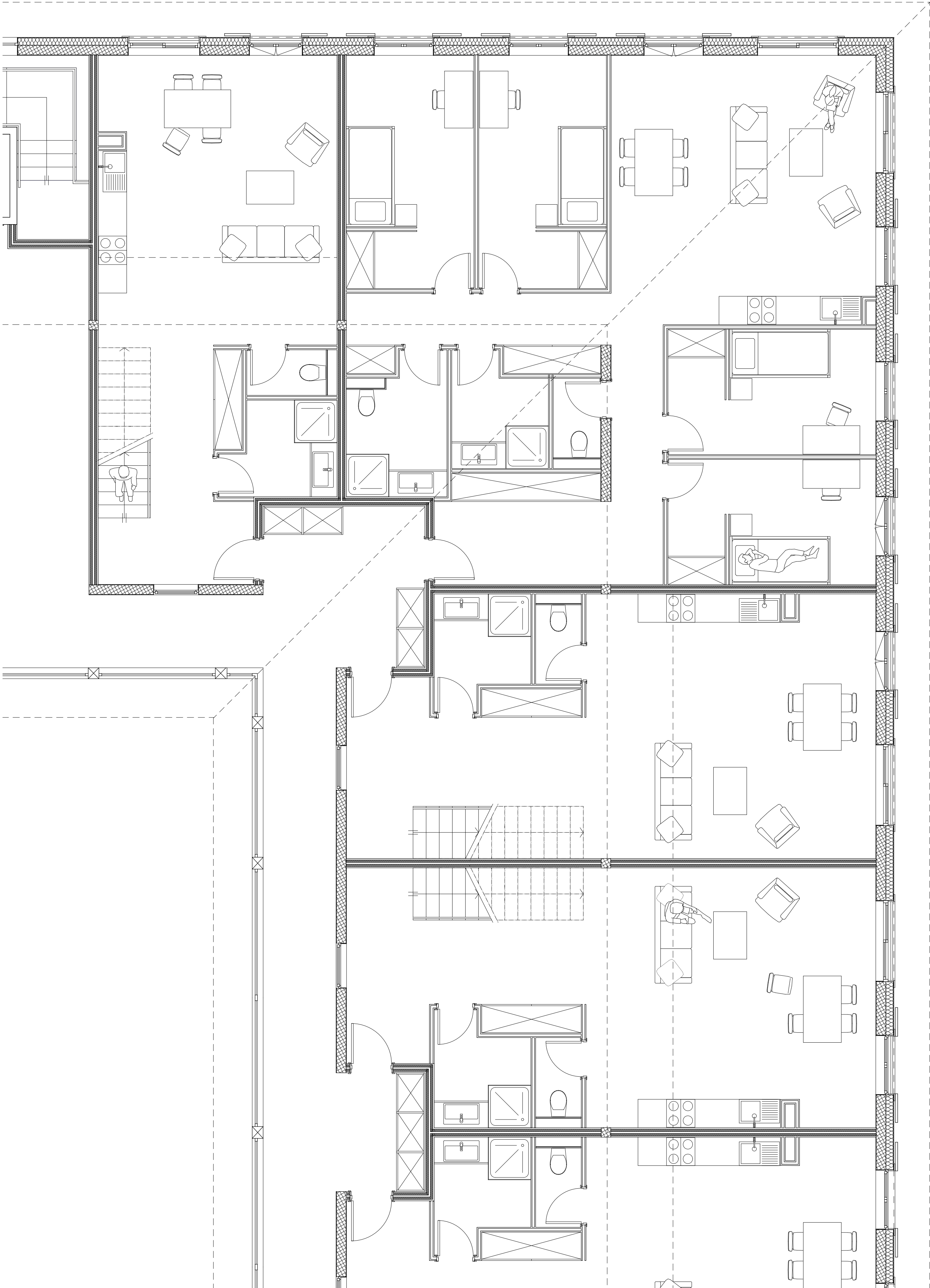
PLAN ÉTAGE COMBLE E 1:50
