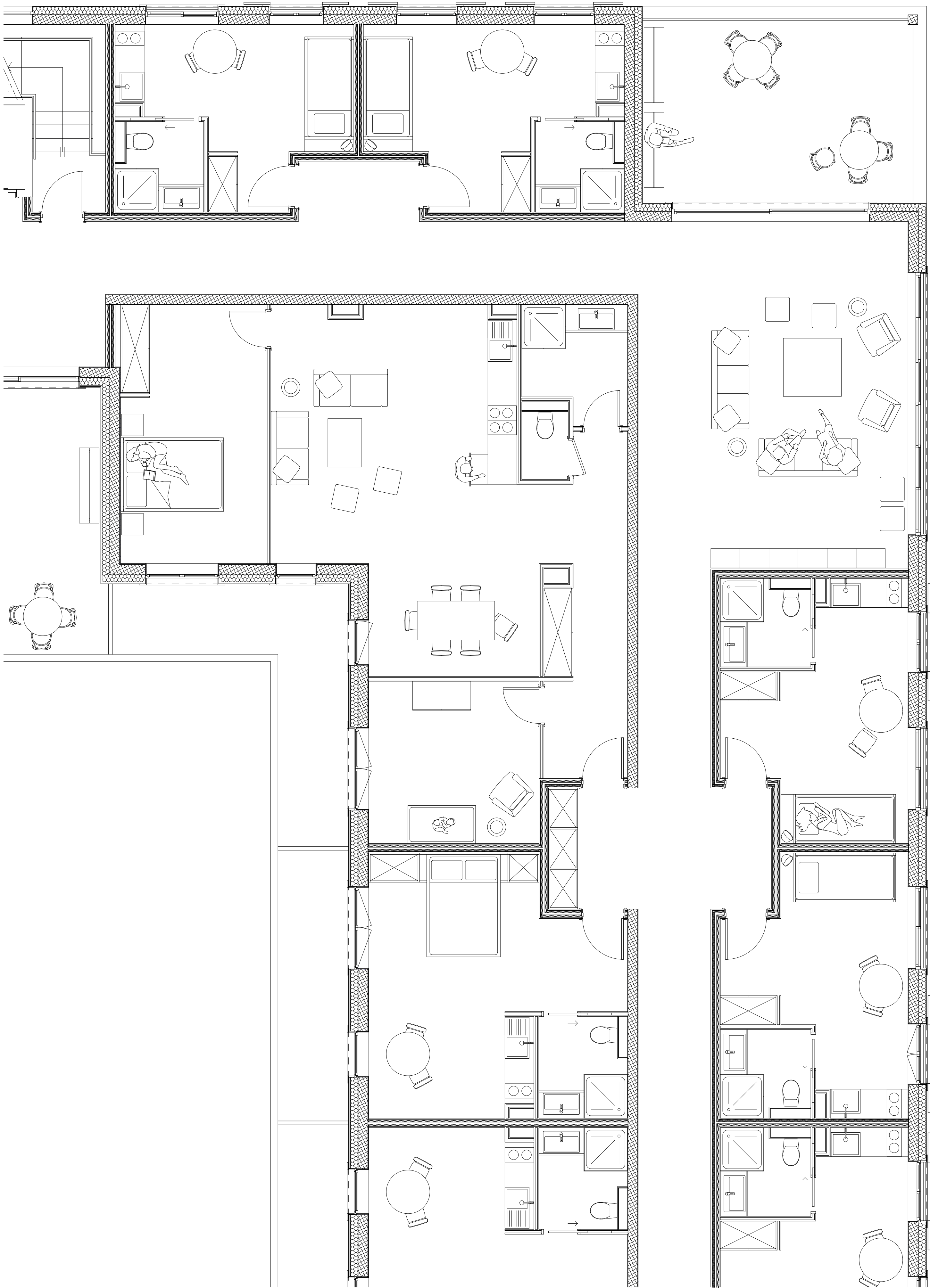
PLAN ÉTAGE TYPE E 1:50
