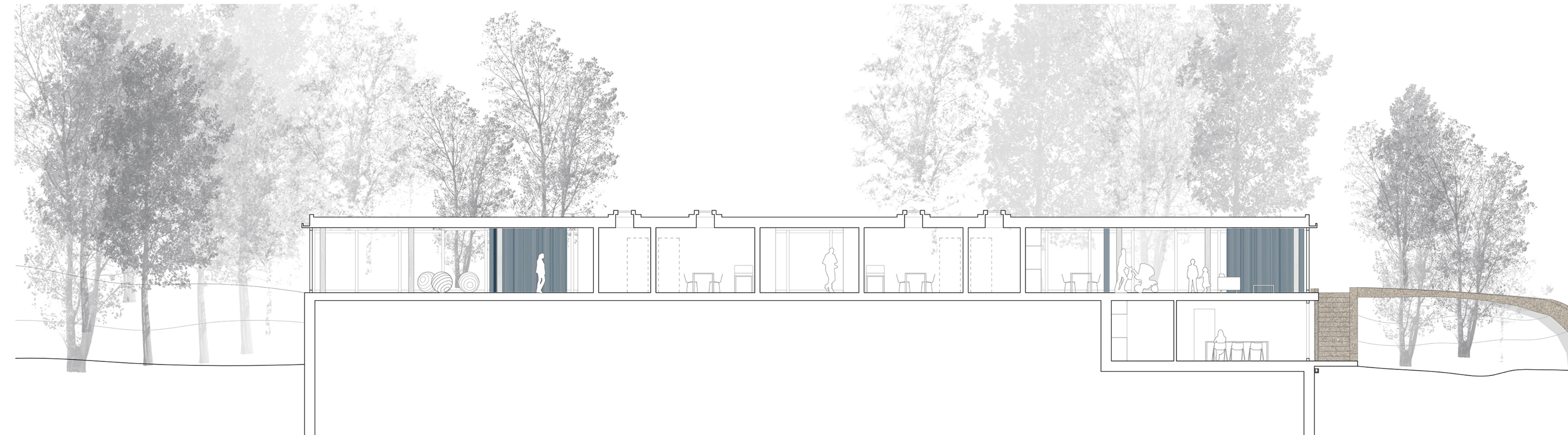
Maison de naissance - coupe longitudinale - 1/100
