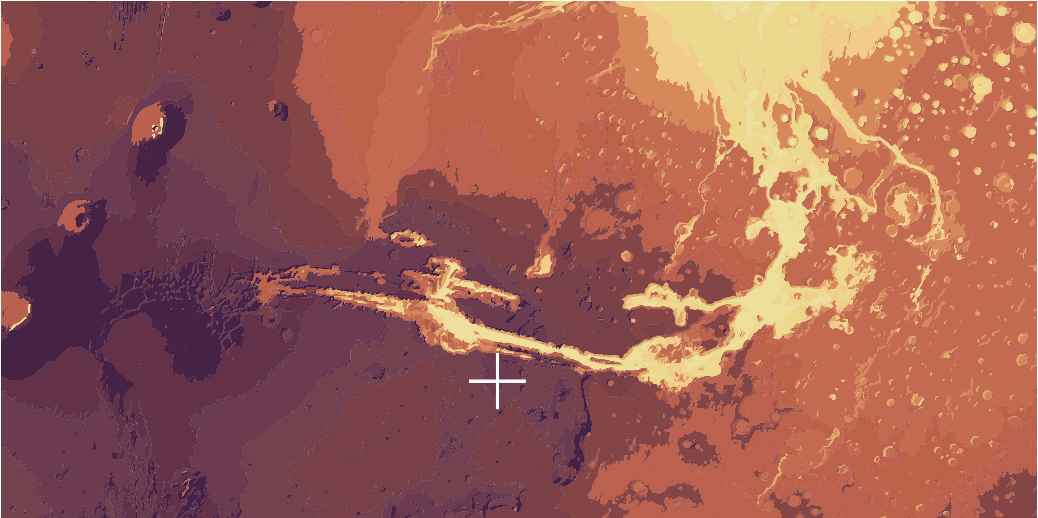
Valles Marineris / Les Vallées de Mariner
