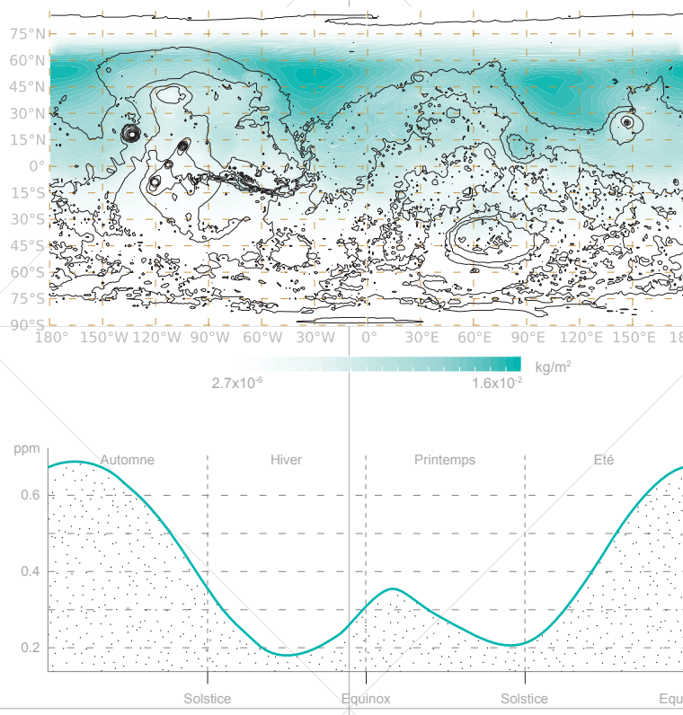
Colonne de vapeur d'eau / Concentration méthanique
