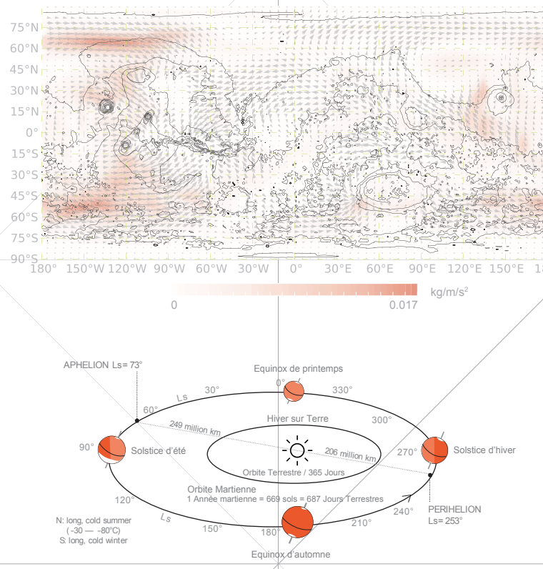
Vents de surface
