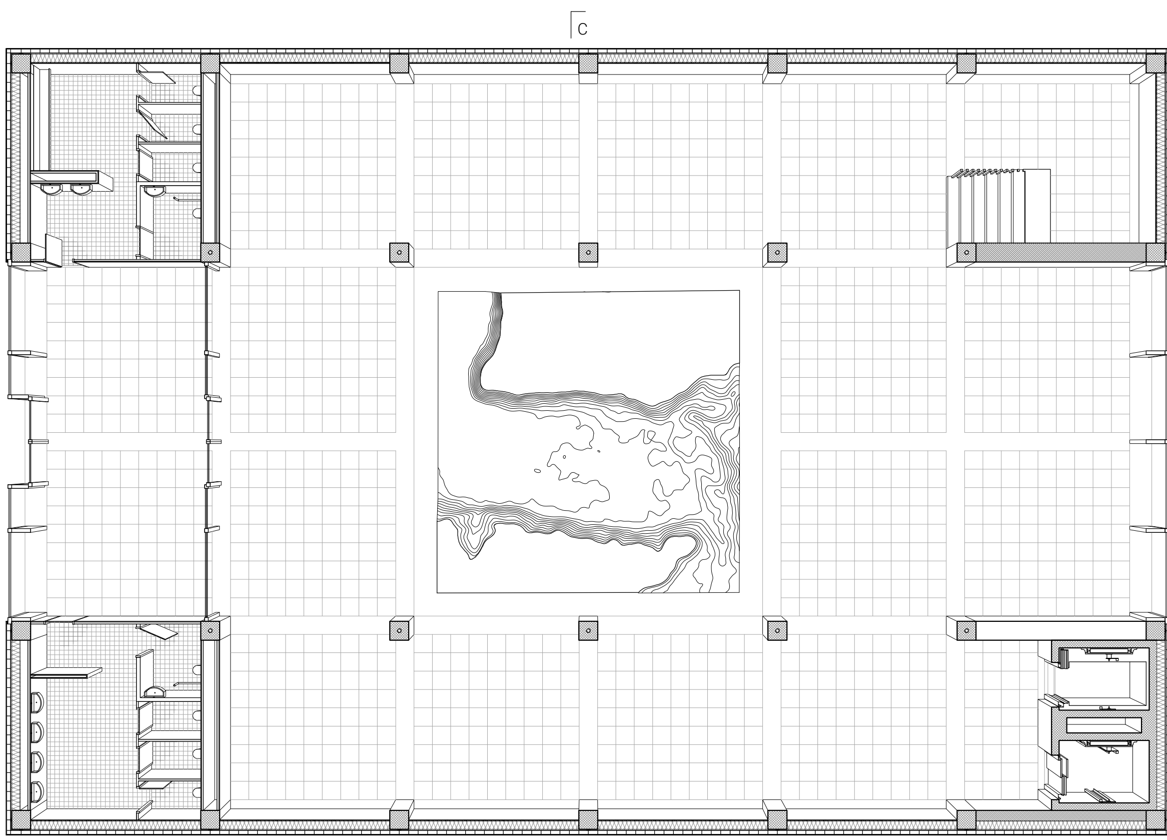
Plan du rez-de-chaussée au 1:100
