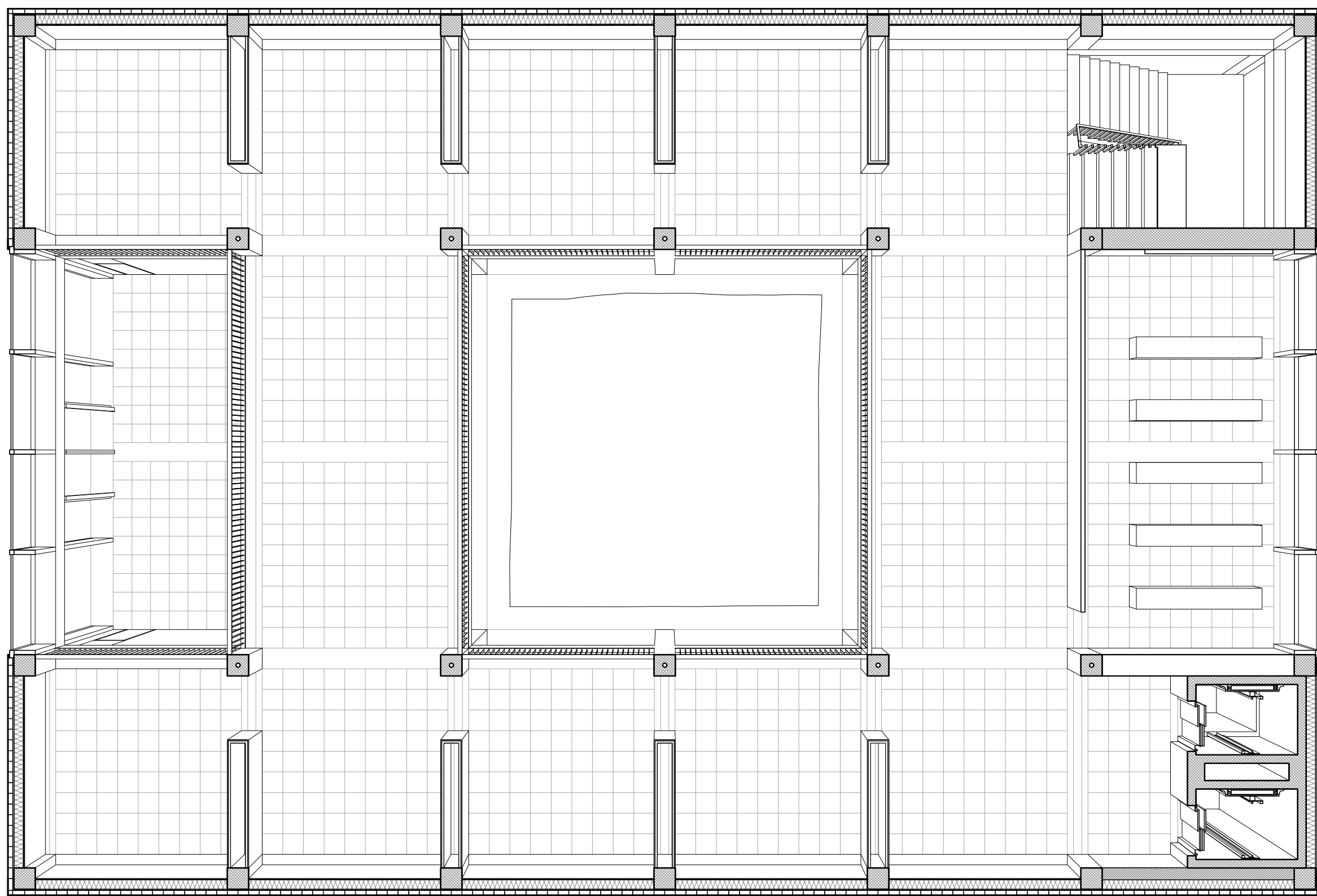
Plan du 1er au 1:100
