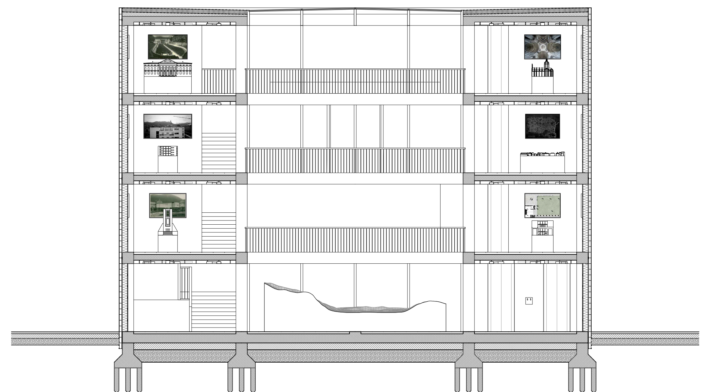
Coupe CC au 1:100
