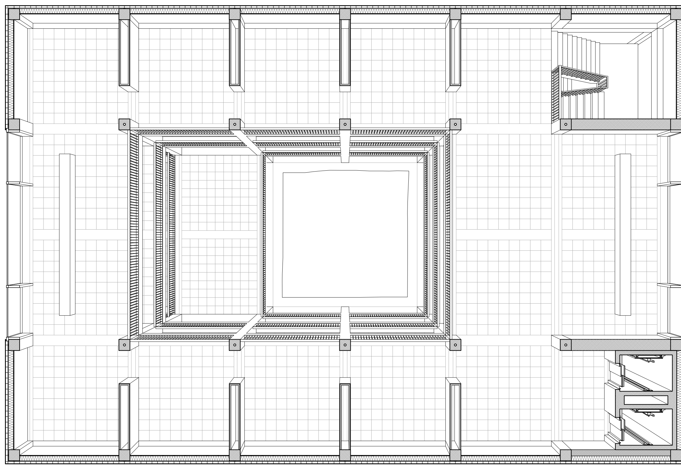
Plan du 3ème au 1:100
