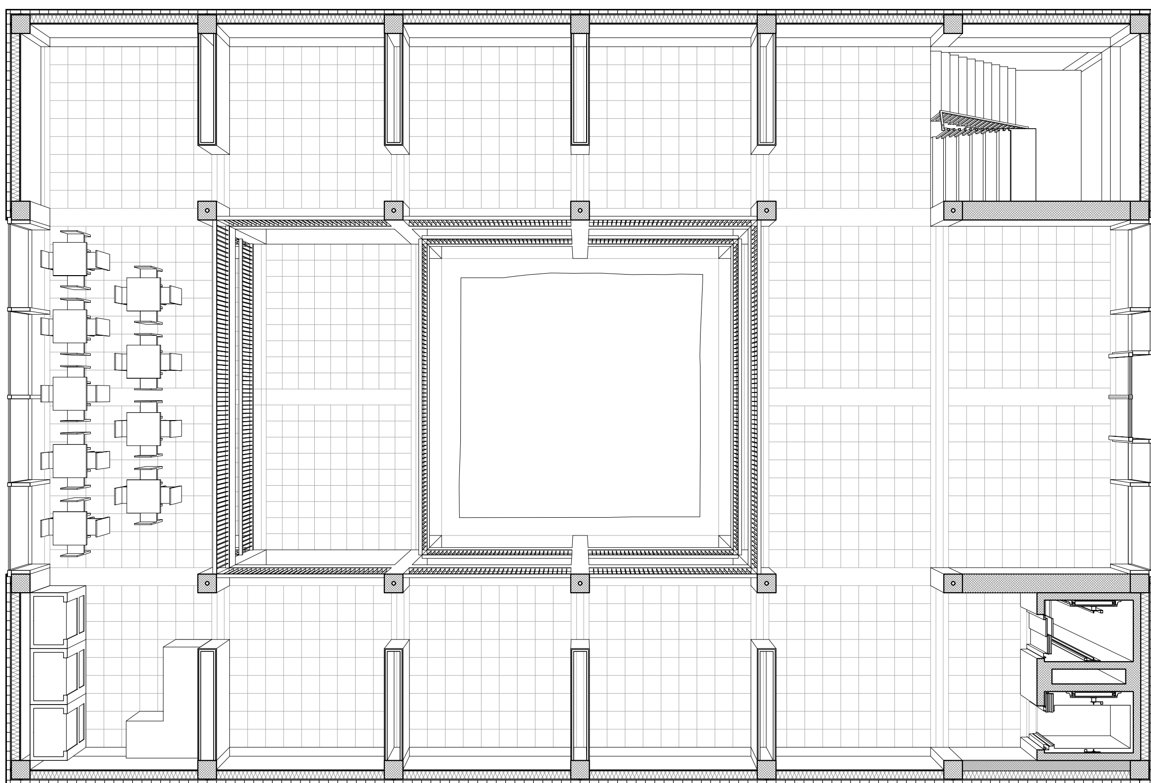
Plan du 2ème au 1:100
