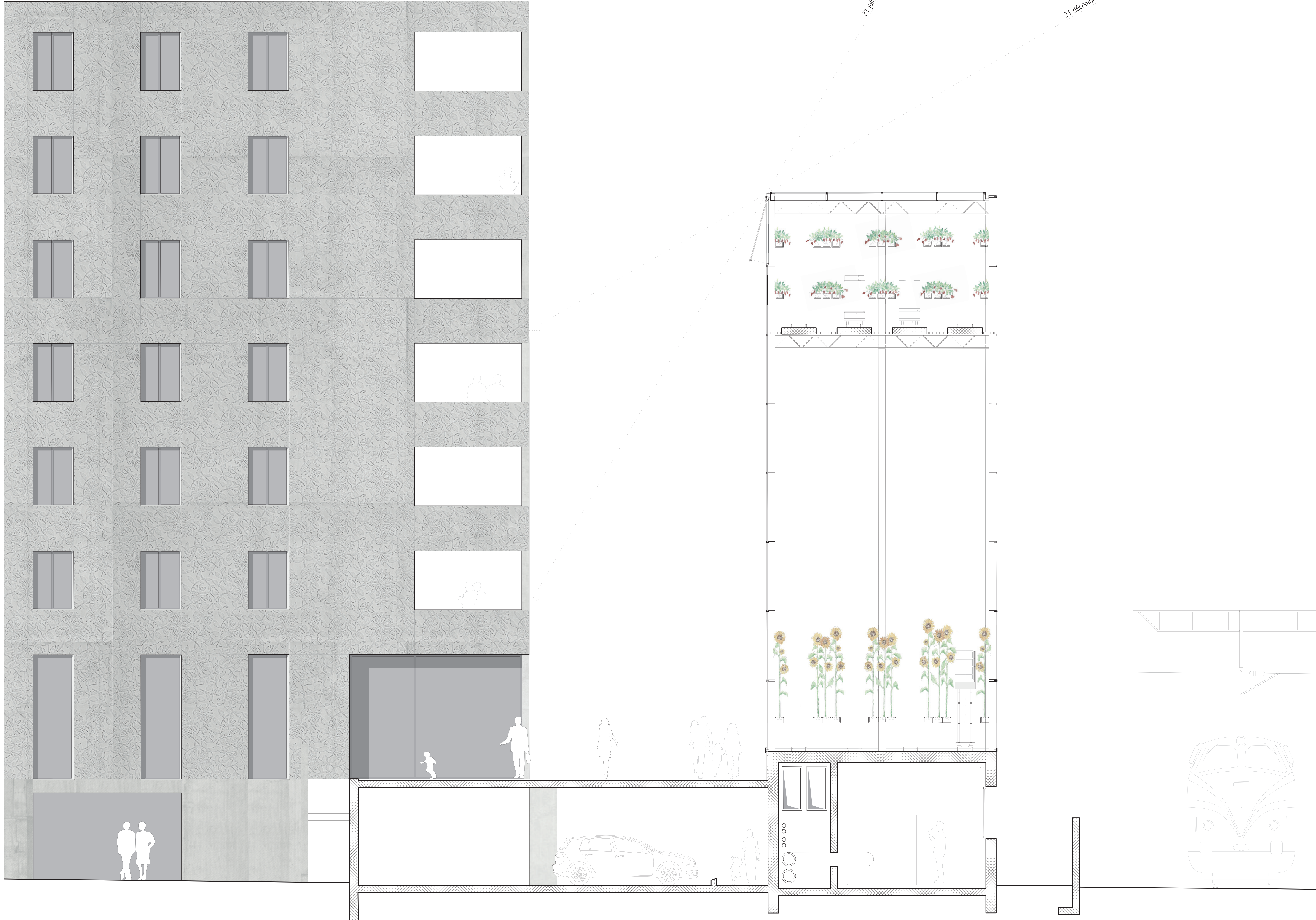
Coupe type _ 1/50
