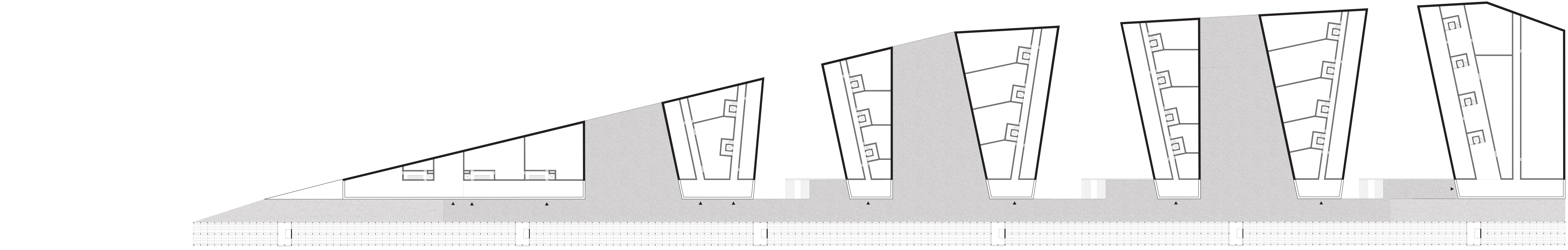
Plan rez inférieur _ 1/500
