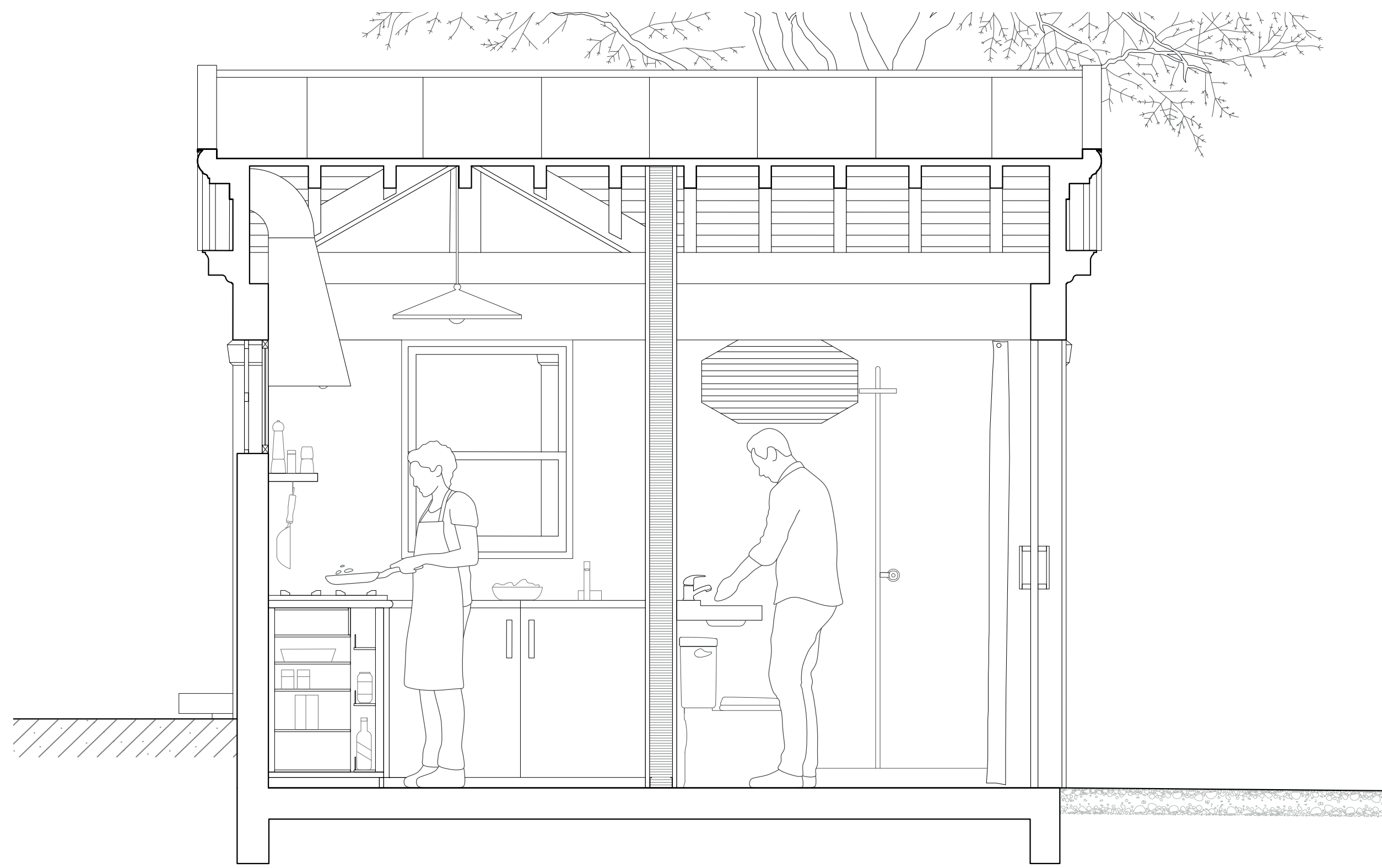
Coupe B - Edicule 1:20
