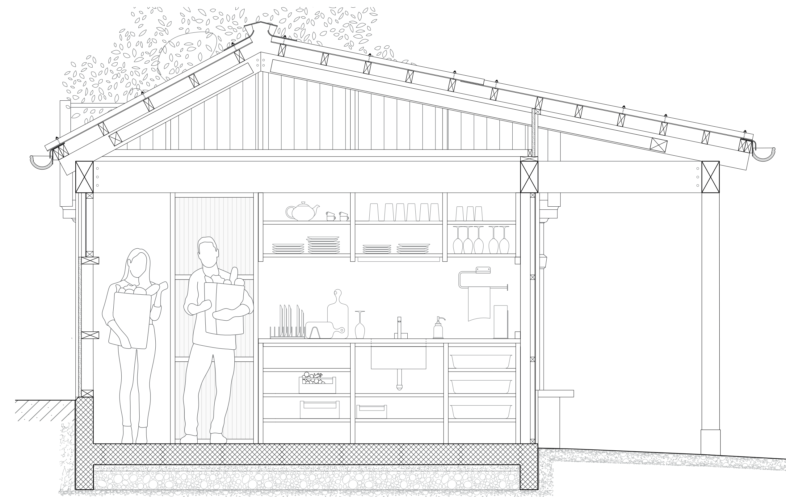
Coupe B' - Pavillon 1:20
