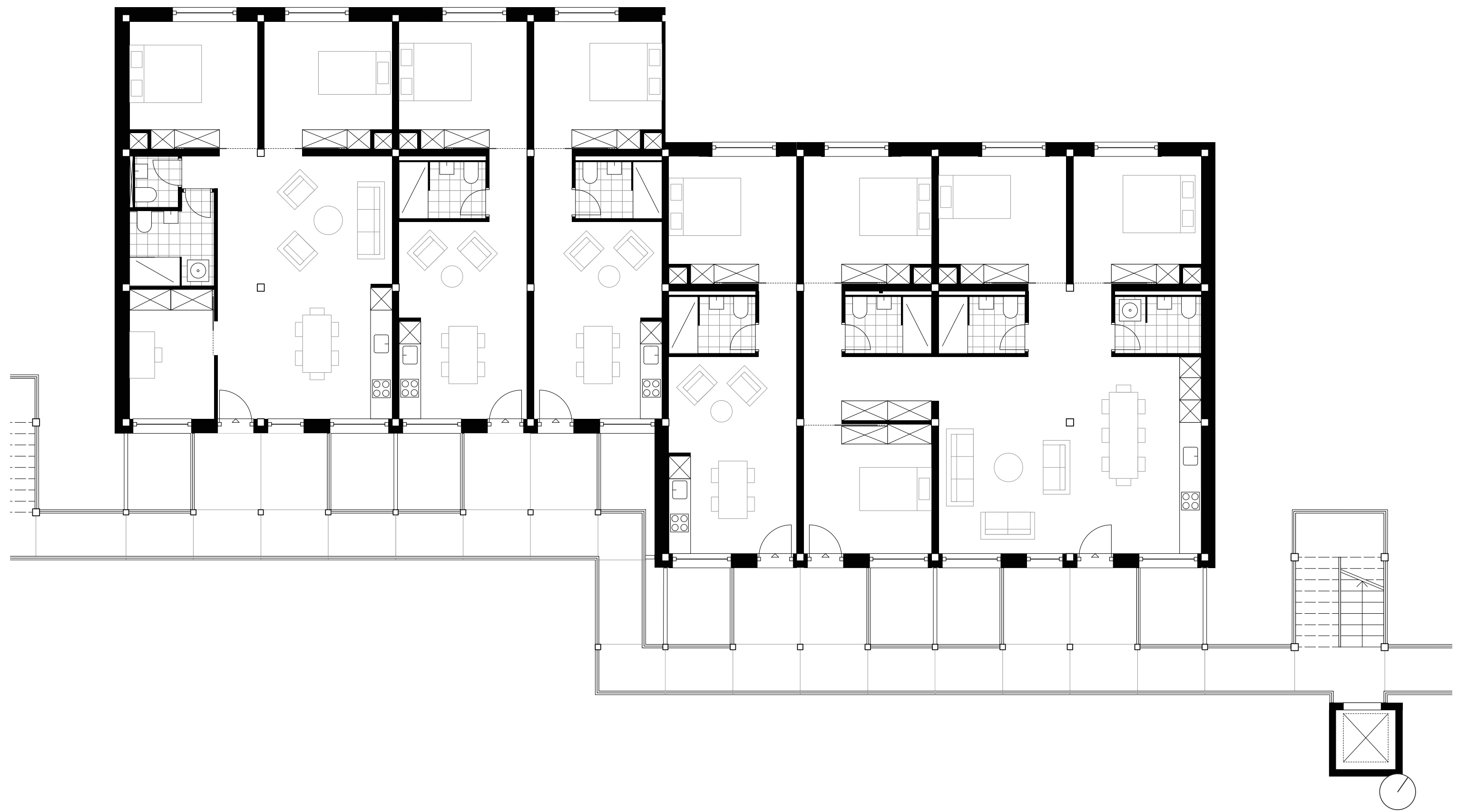
Plan Bâtiment HAUT (NORD) 1:100
