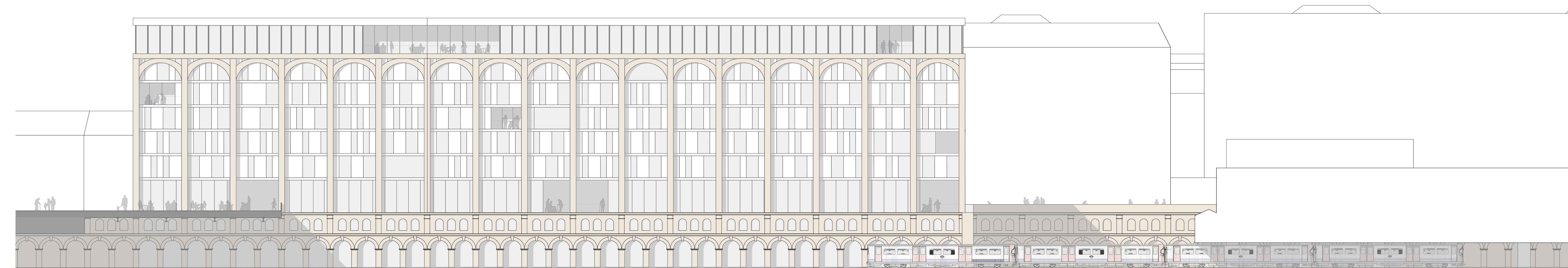
Elévation sur quais 1/500
