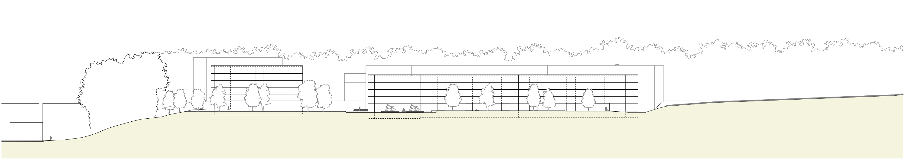
Coupe longitudinale bb - 1:1000
