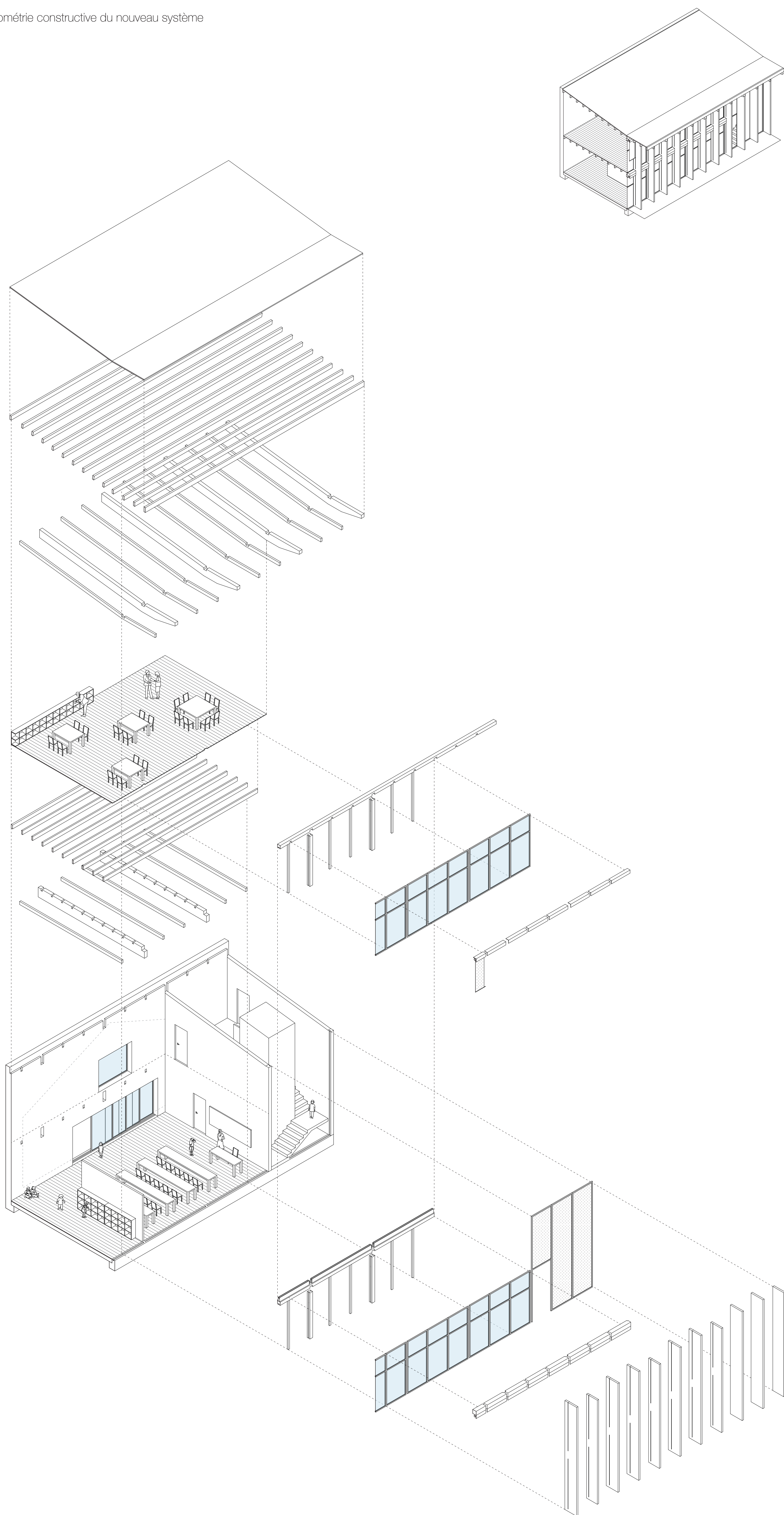
Axonométrie constructive du nouveau système
