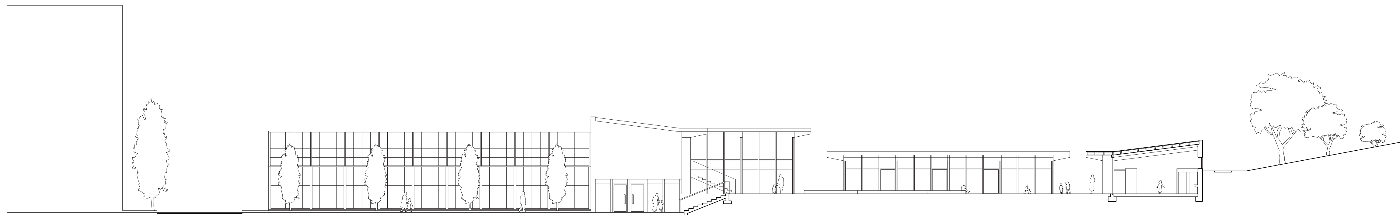
Coupe transversale BB' 1/200
