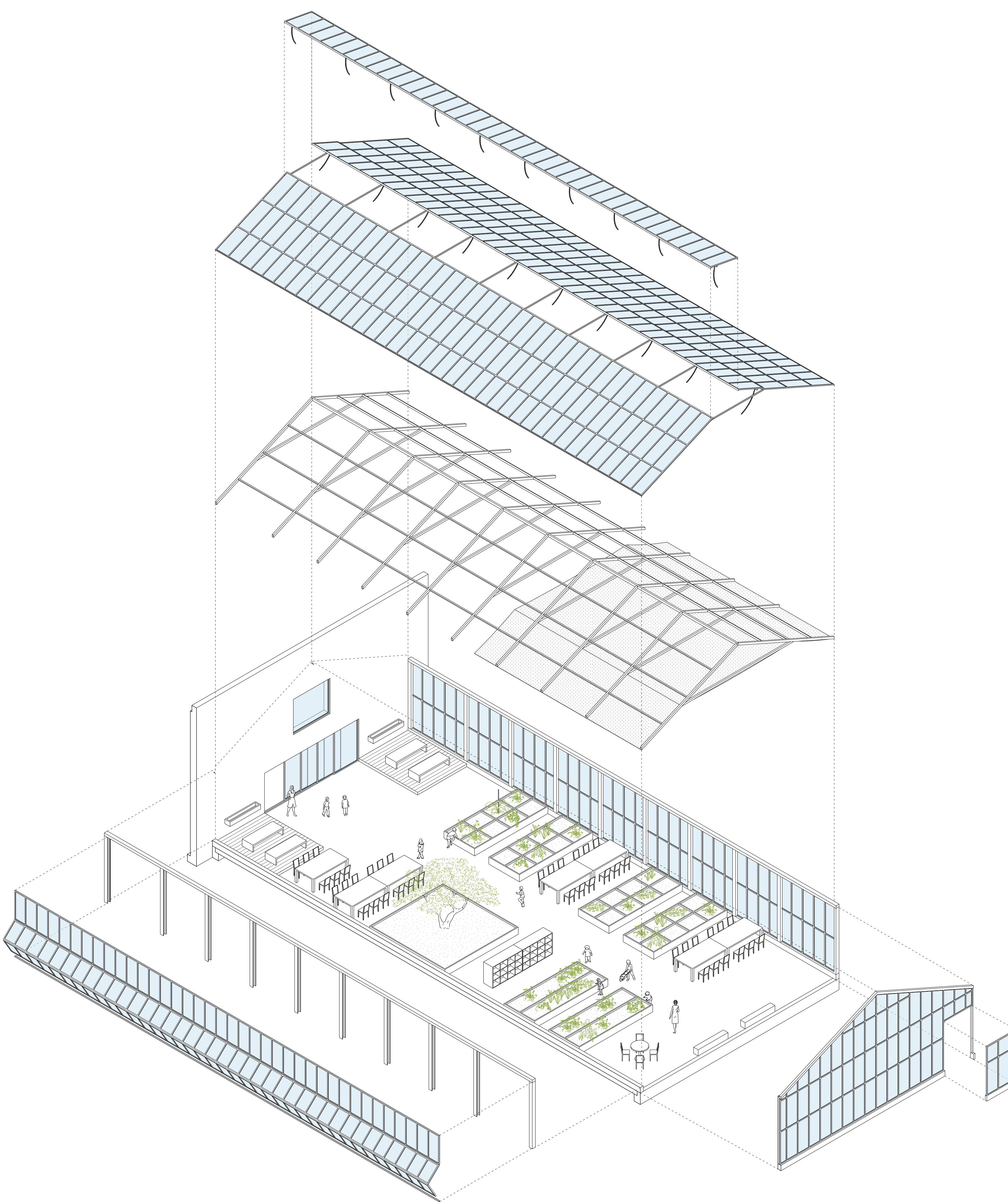
Axonométrie constructive d'une unité de serre
