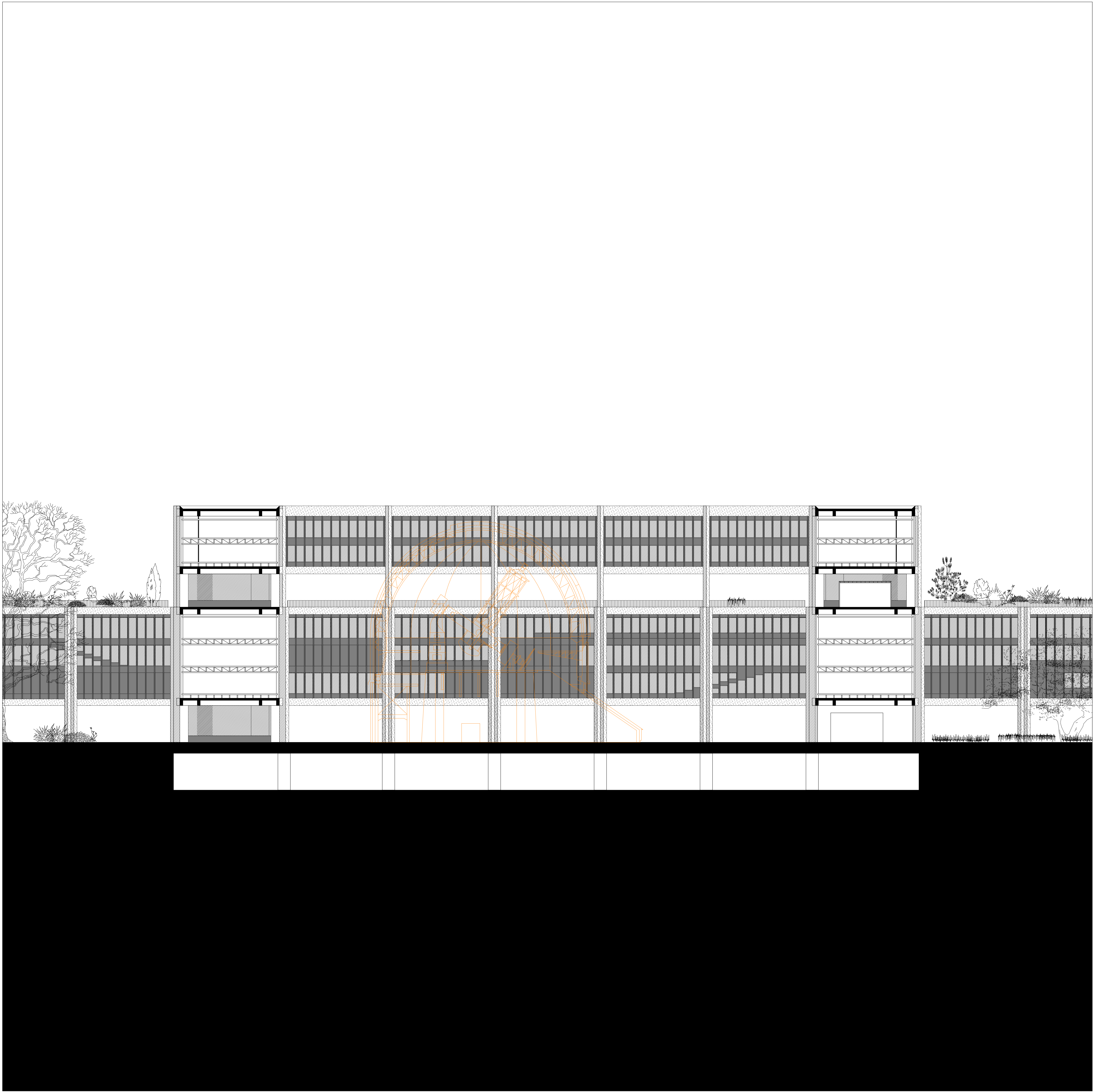
Coupe - 1:200
