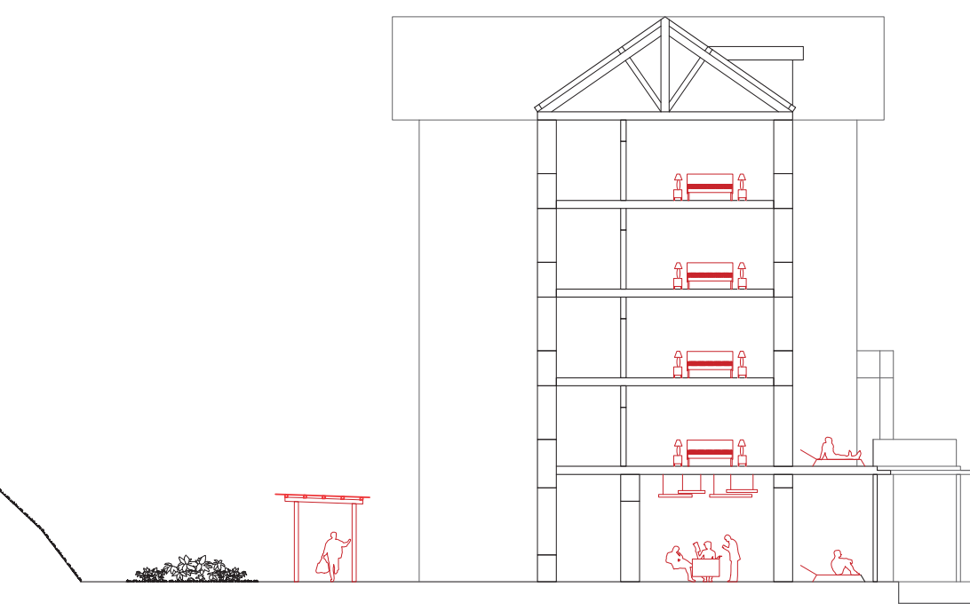
HÔTEL POUR SENIORS COUPE - 1:250
