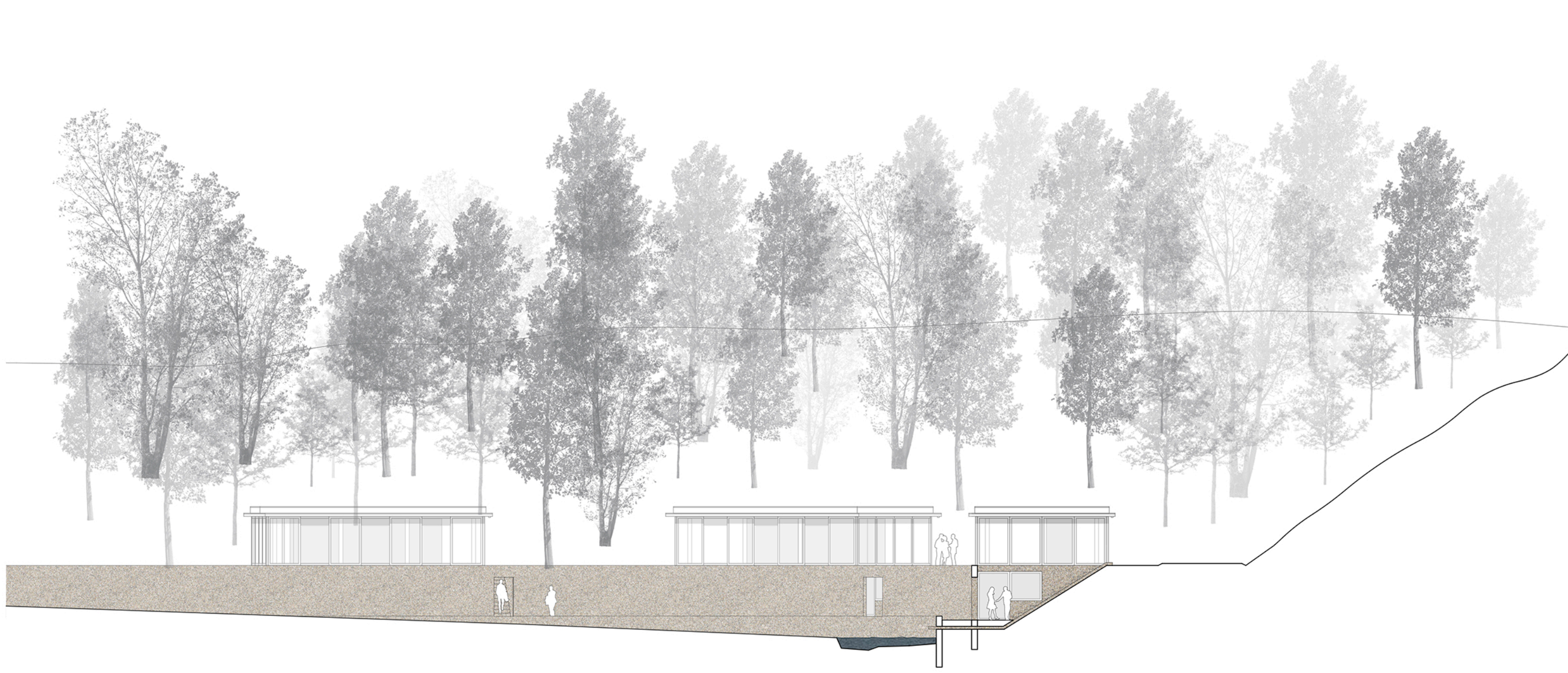
Parcours - coupe BB - 1/200
