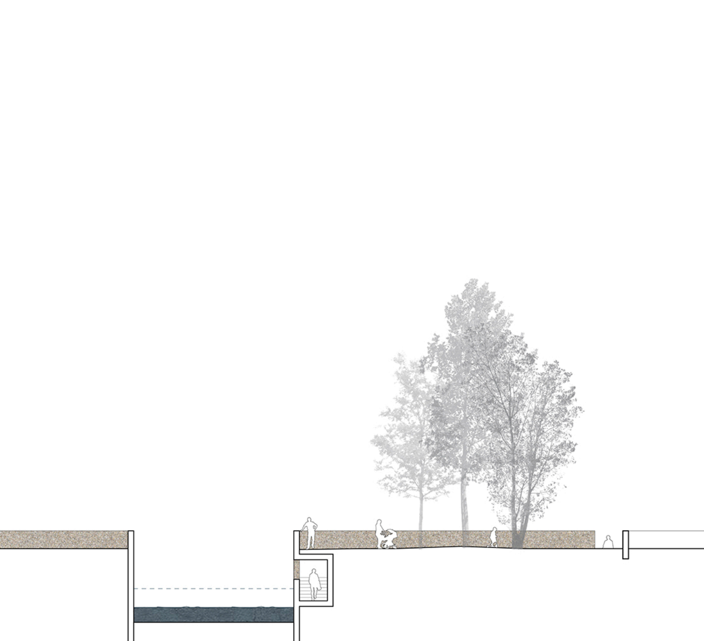
Parcours - coupe EE - 1/200
