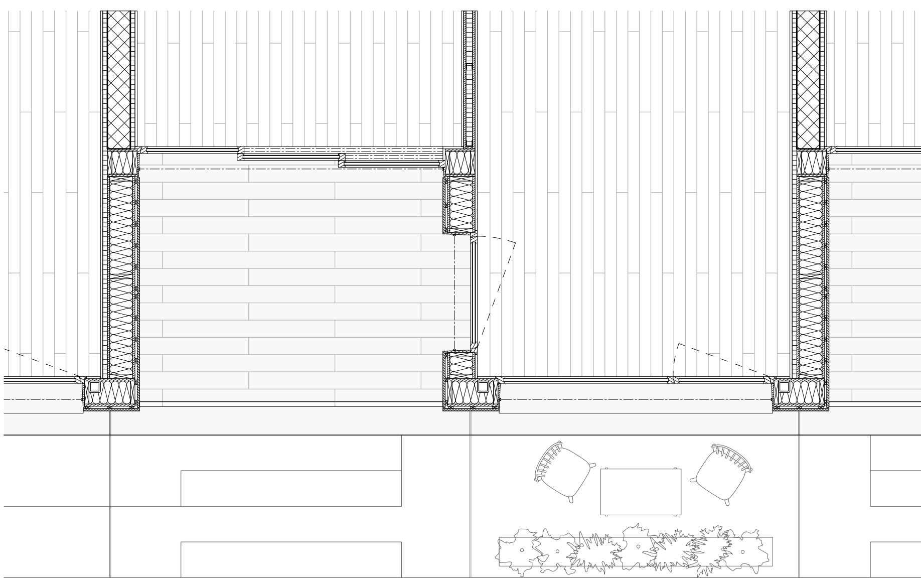
Plan, coupe et élévation de l'enveloppe extérieure 1:33
