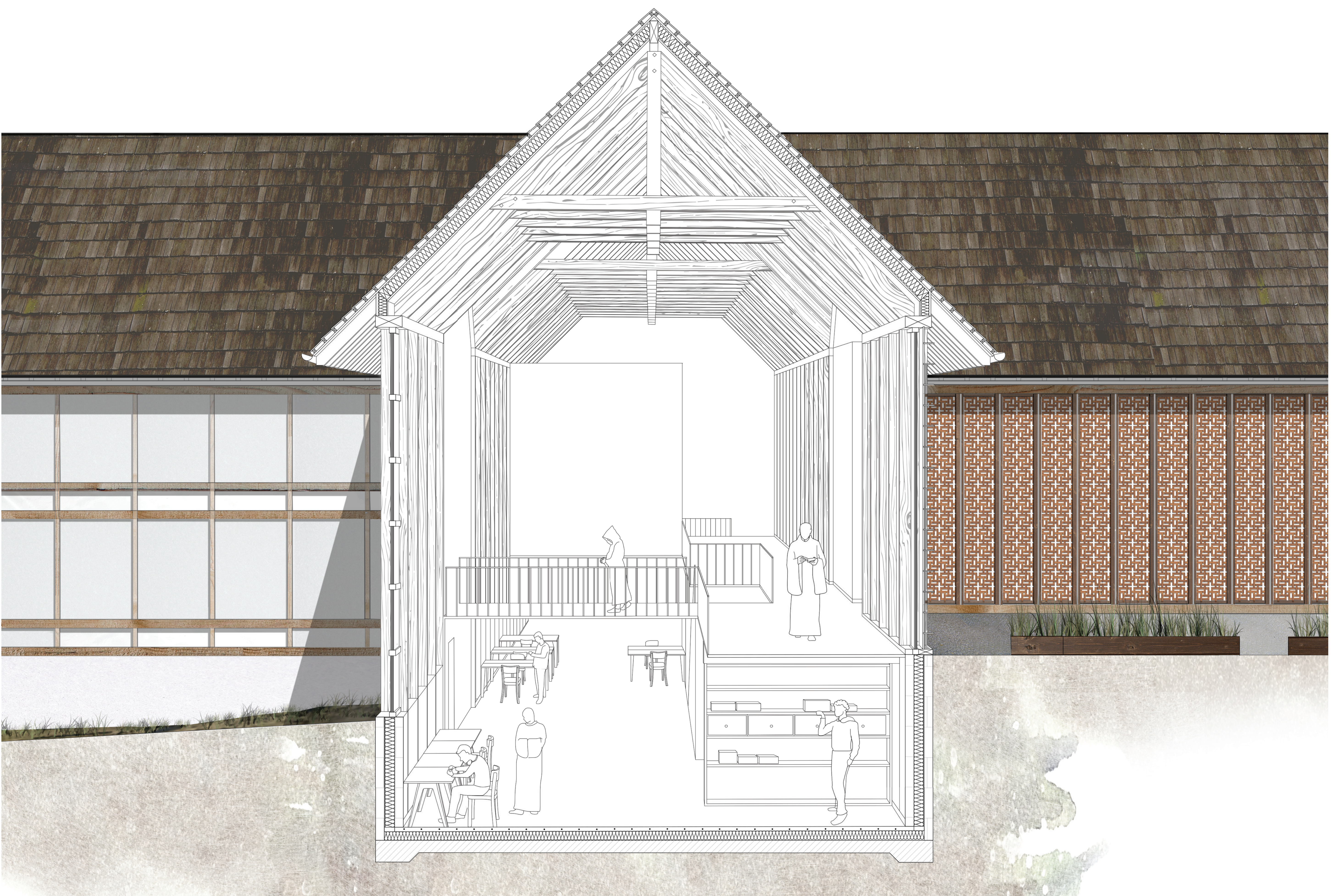
Coupe perspective constructive 1:33
