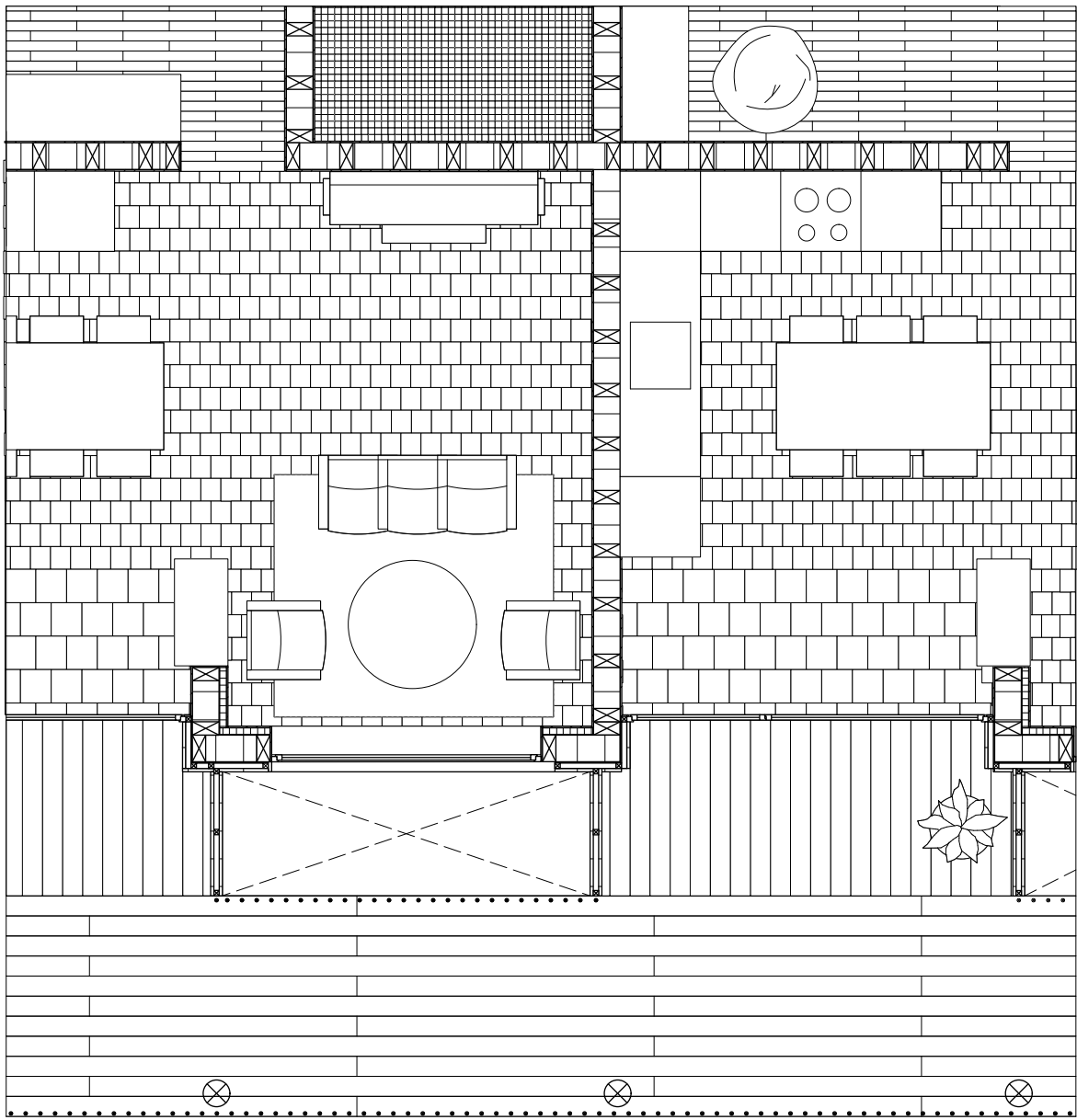
Détail plan 1:50
