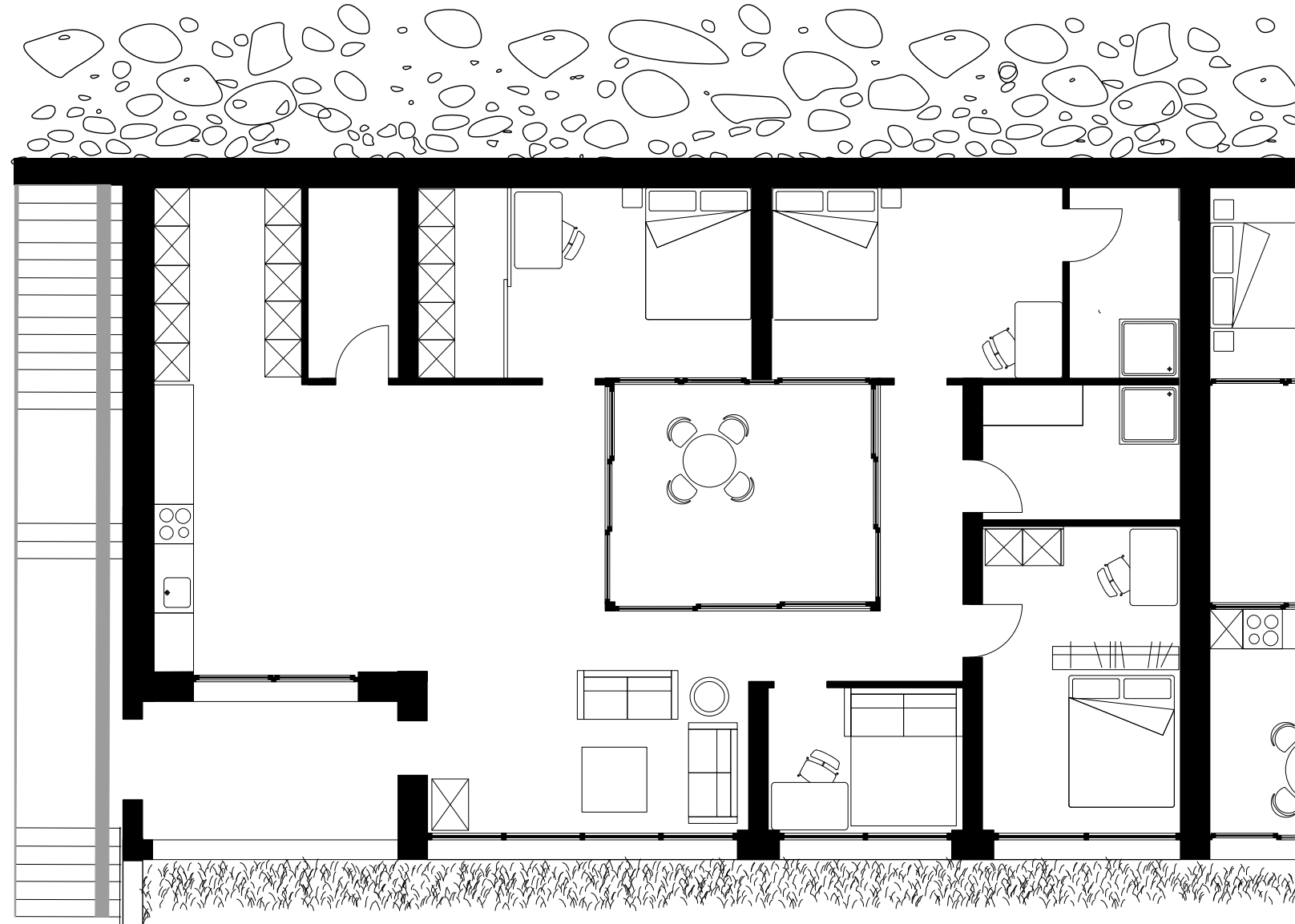
Typologie + Coupe-élévation grand appartement 1:100
