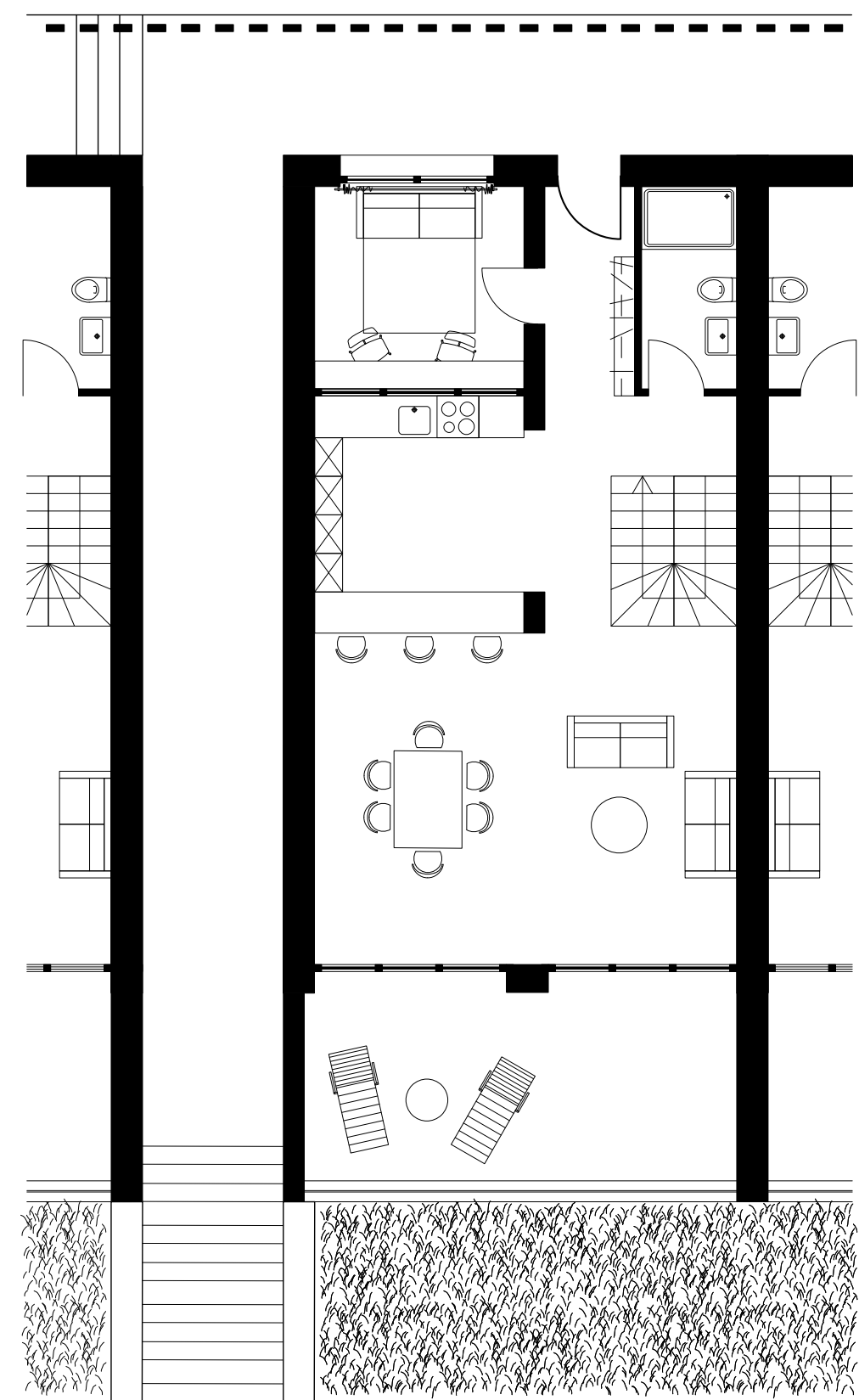
Typologie + Coupe-élévation duplex 1:100
