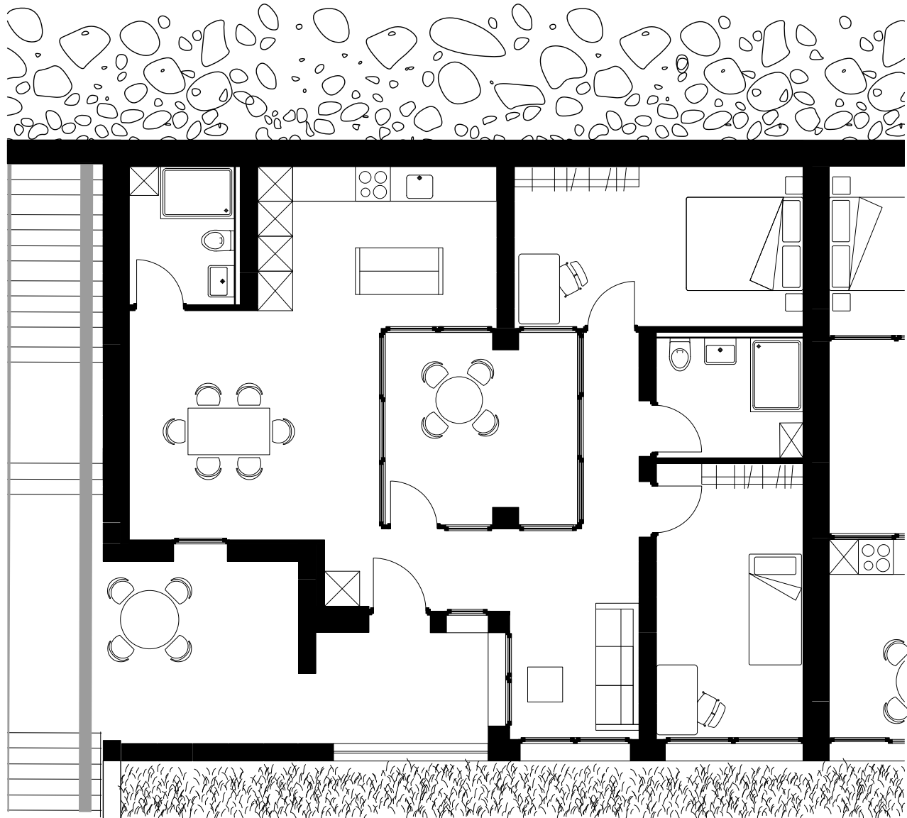
Typologie + Coupe-élévation appartement moyen 1:100
