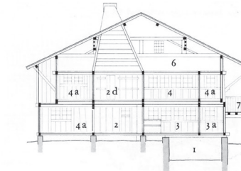
629 Coupe transversale A-A 1:200
