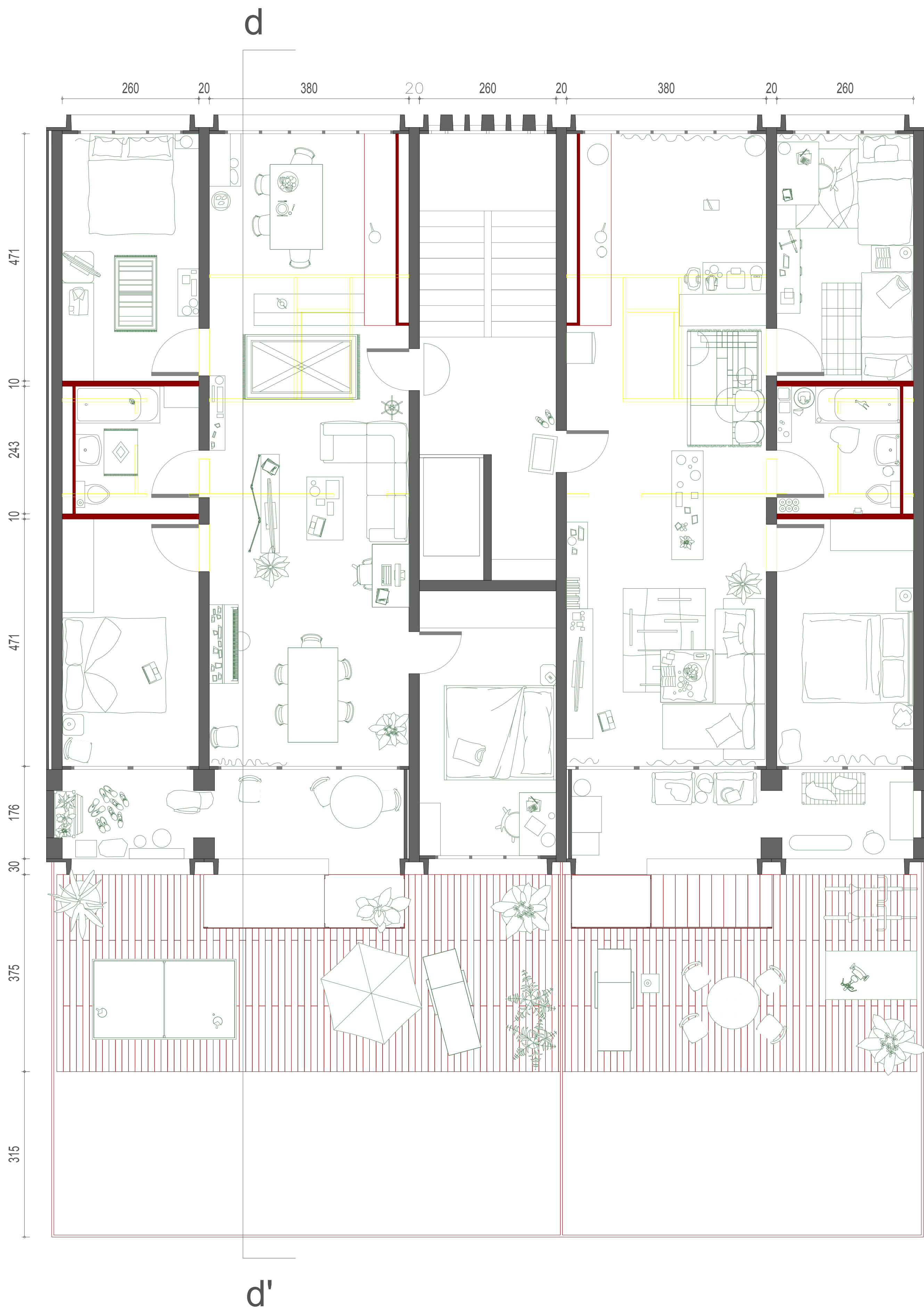
Plan d'un étage existant, ajout d'un accès au jardin privé et modification des parois non porteuses
