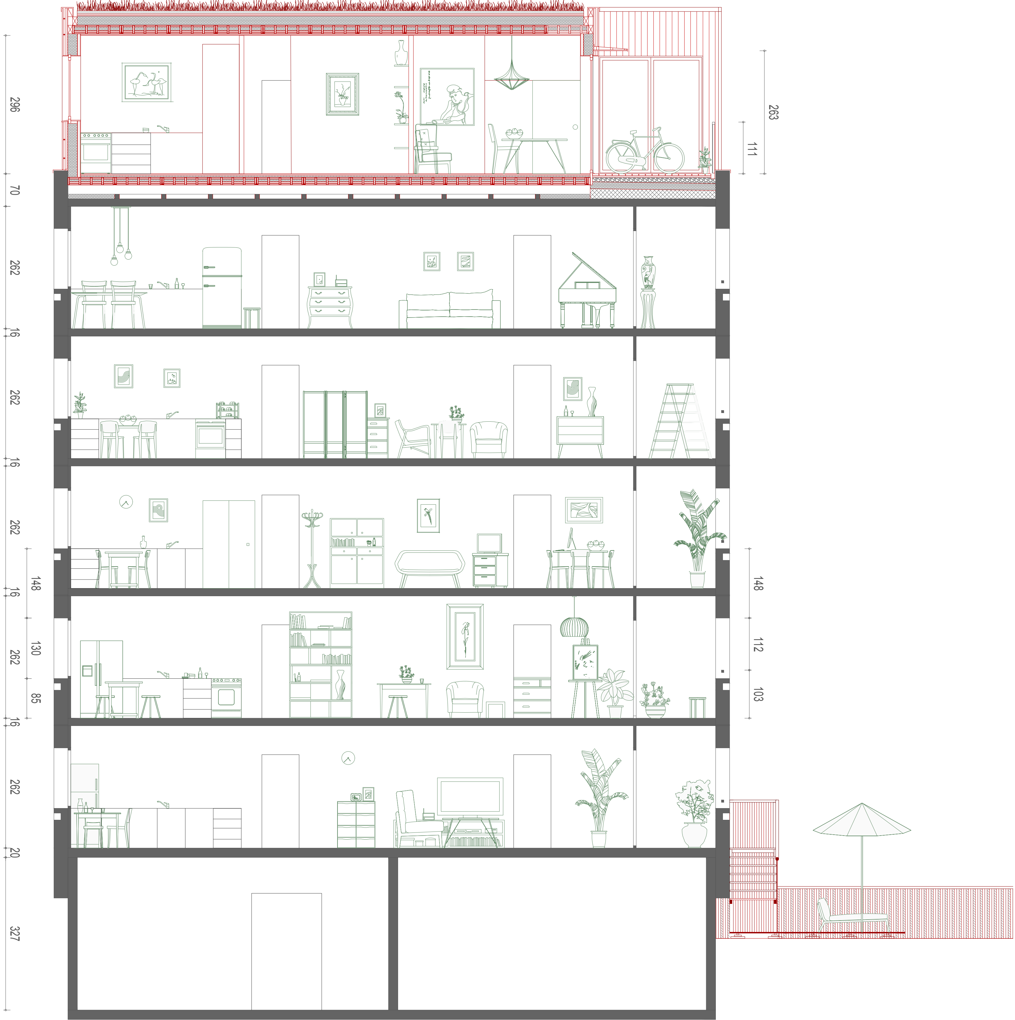
Coupe d'un immeuble type avec sa surélévation
