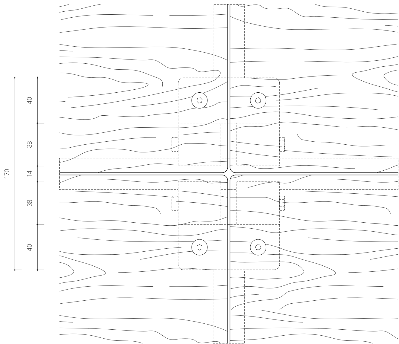
Plan Plancher
