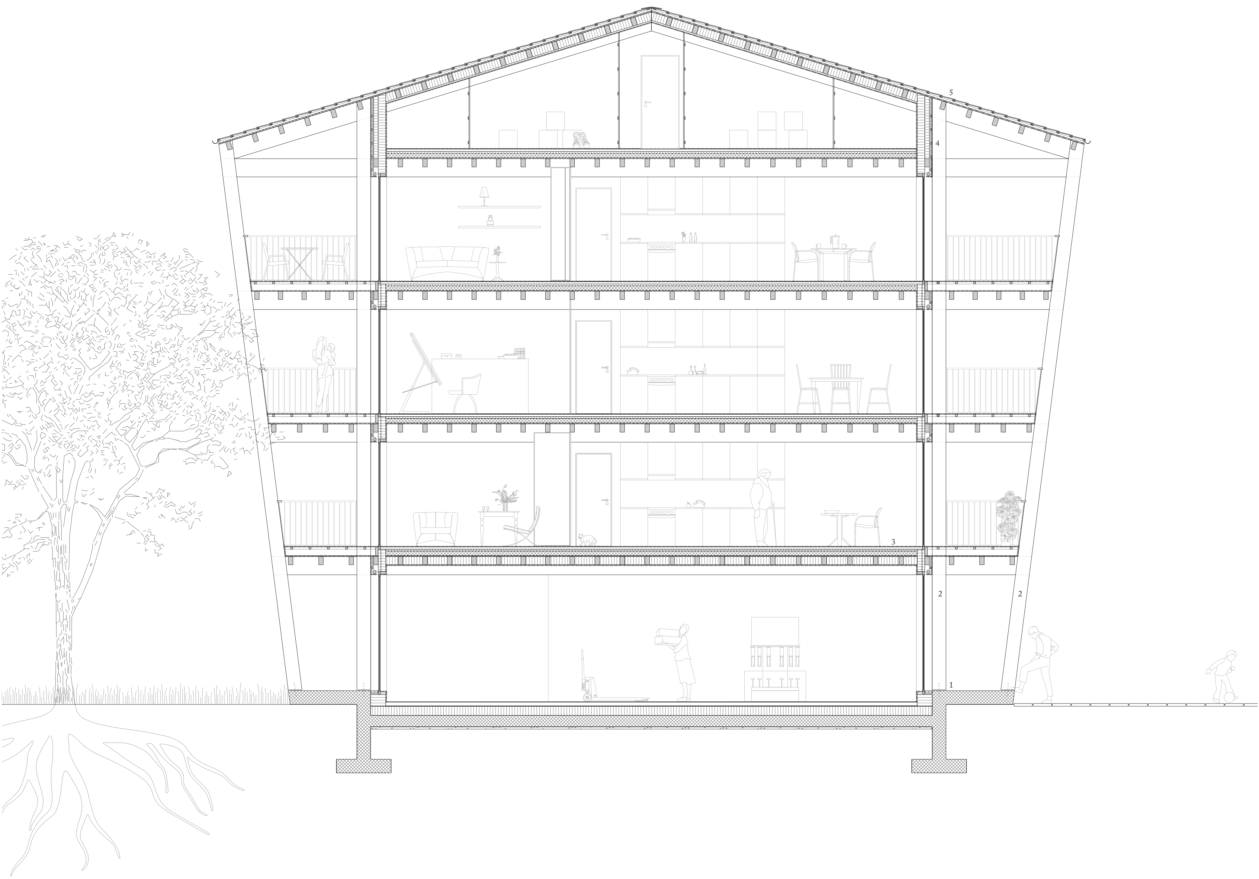
Coupe transversale
